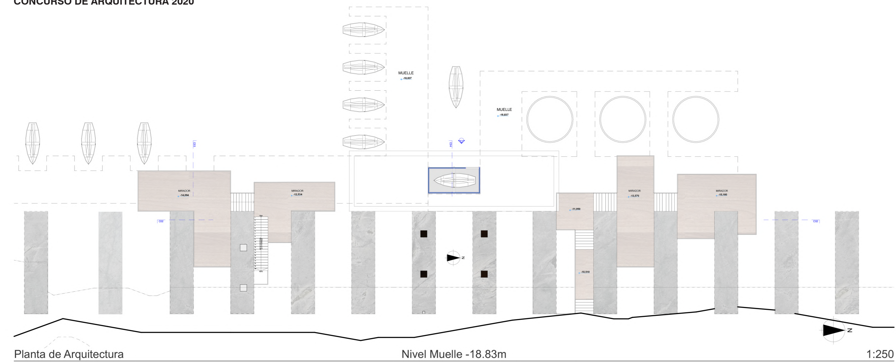
Planta de Arquitectura Nivel Muelle -18.83m 1:250
