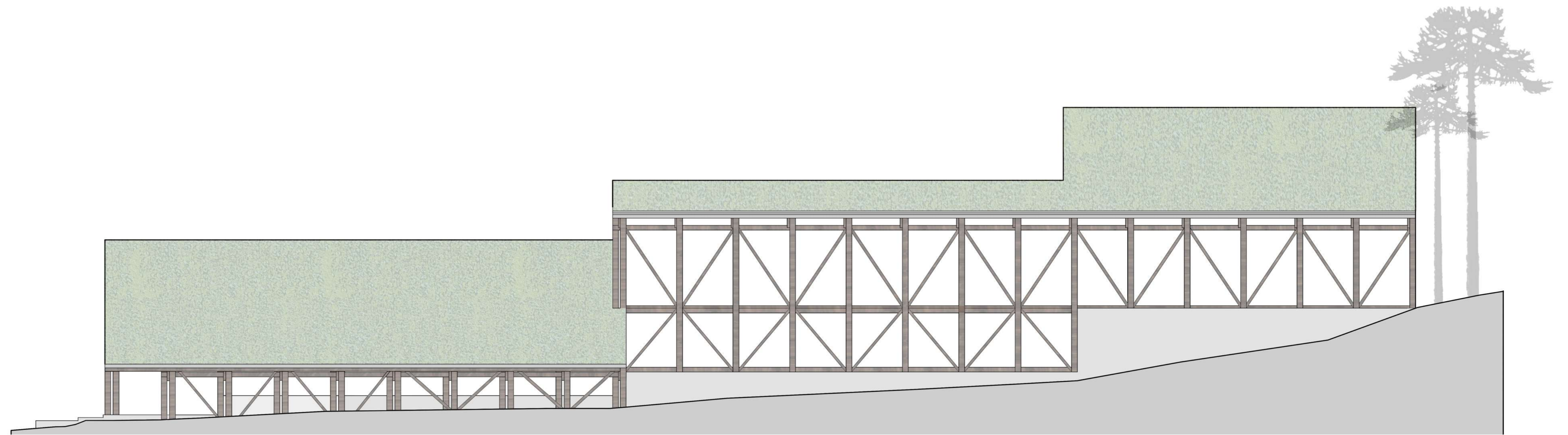
ELEVACIÓN LATERAL ESC 1:100
