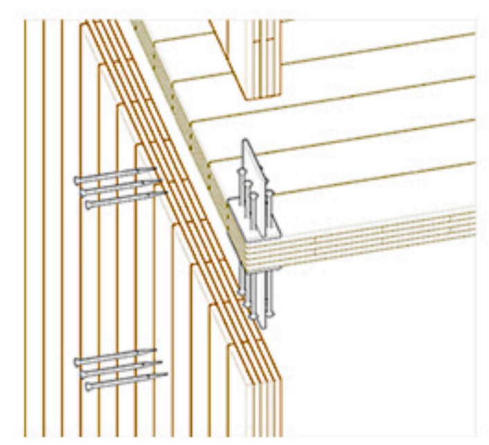
UNIONES PARA SISTEMA DE MUROS Y LOSA CLT
