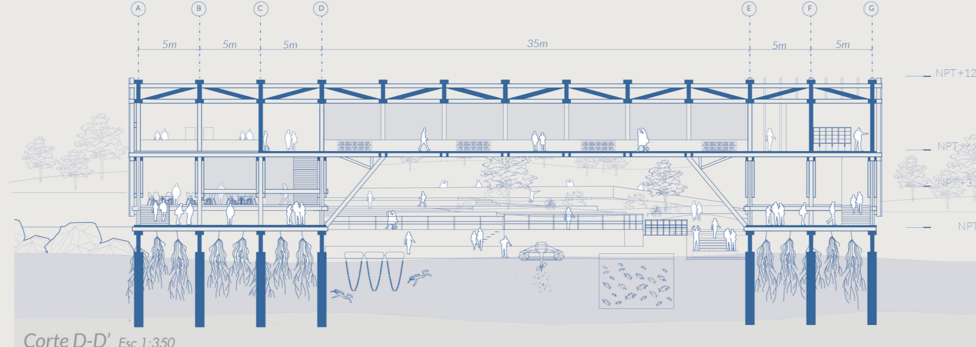
Corte D-D' Esc 1:350
