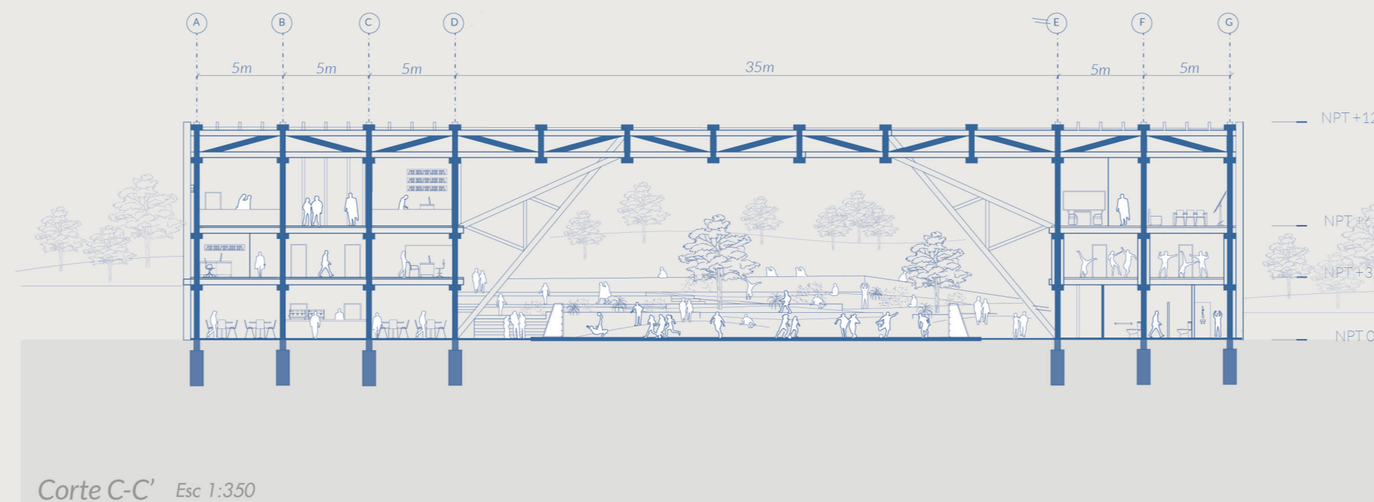
Corte C-C' Esc 1:350
