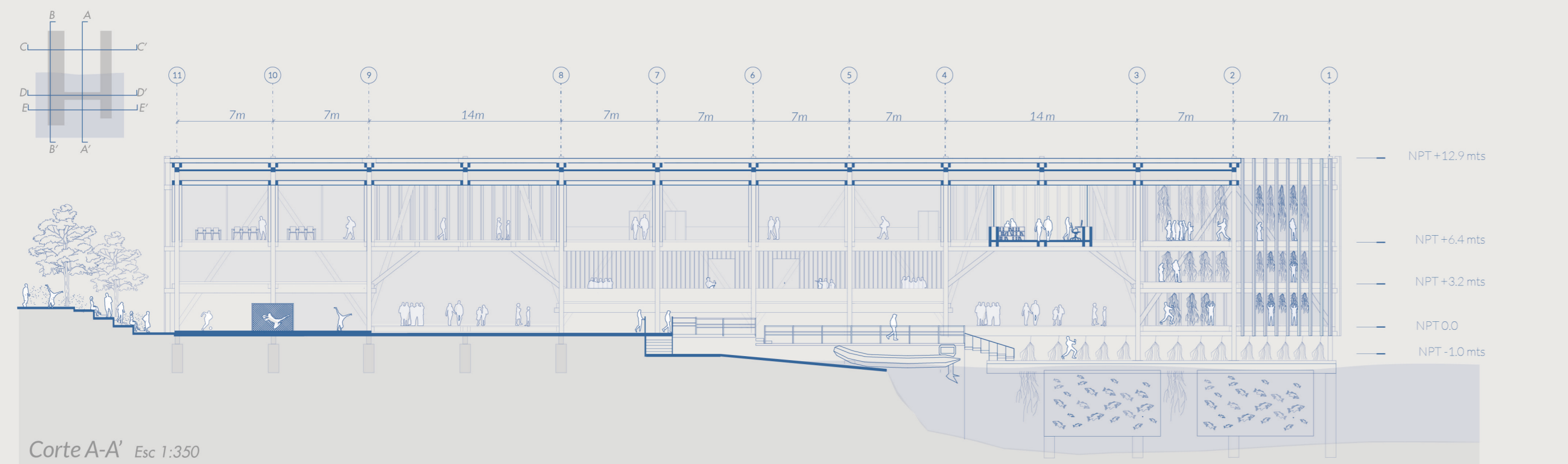
Corte A-A' Esc 1:350
