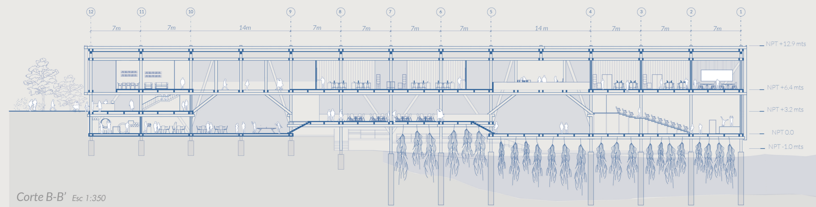
Corte B-B' Esc 1:350
