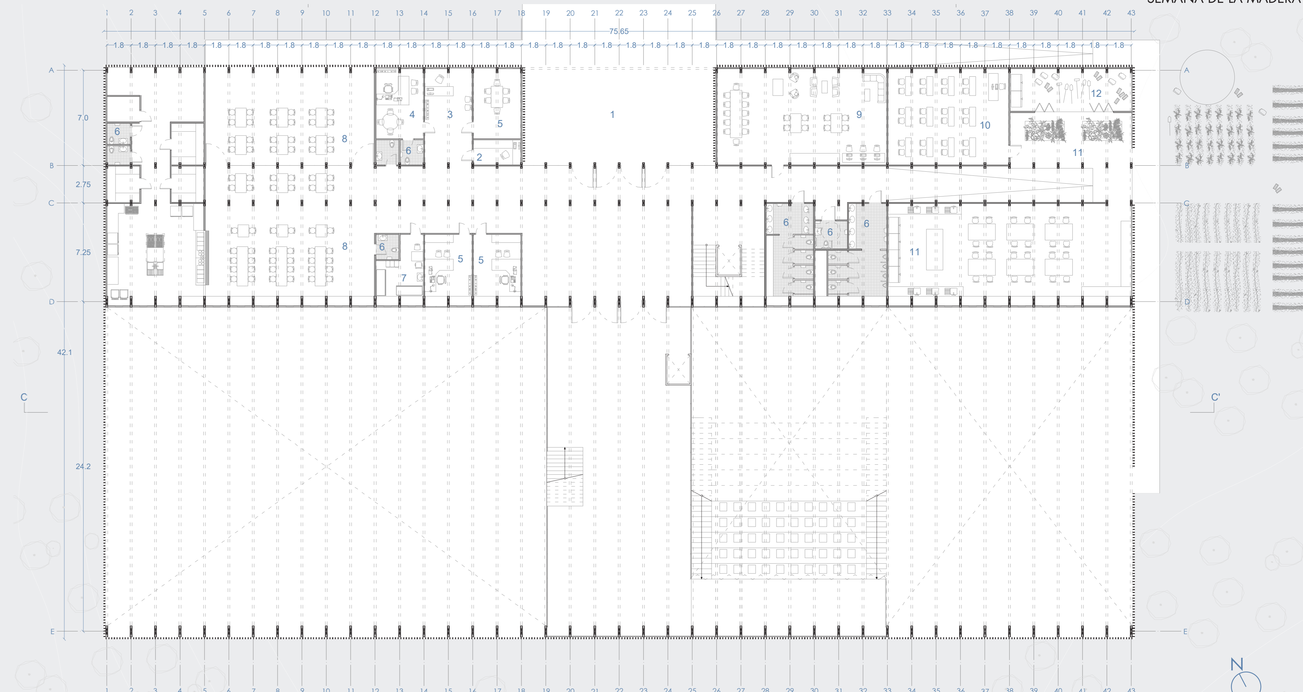
PLANTA NIVEL 1 ESCALA 1/200
