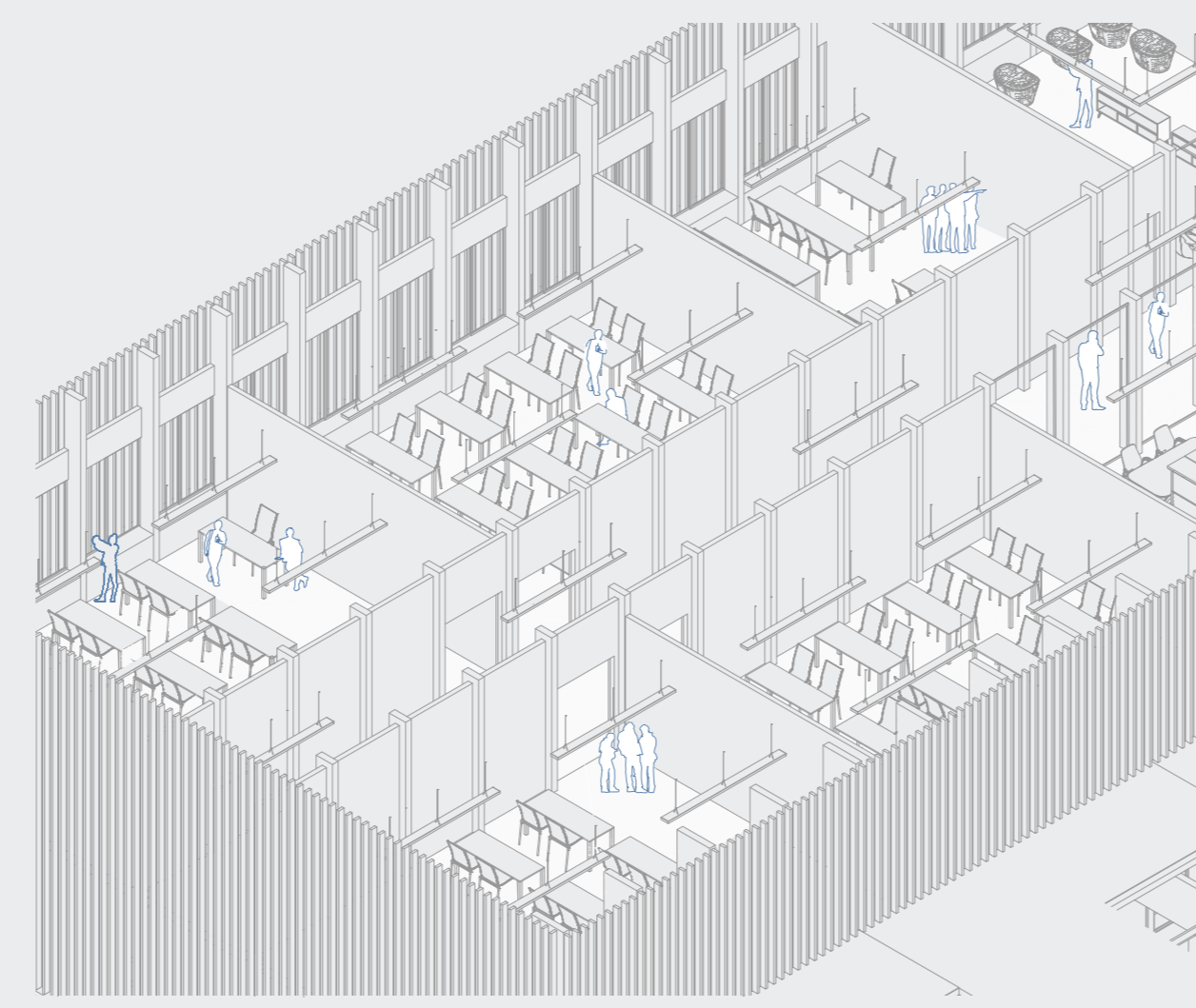
VISTA ISOMETRICA 2DO NIVEL TEORICO
