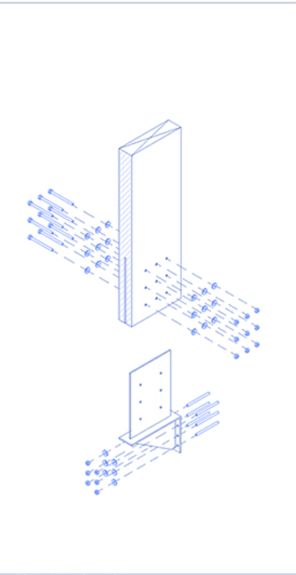
Union Pilar - Losa de suelo
