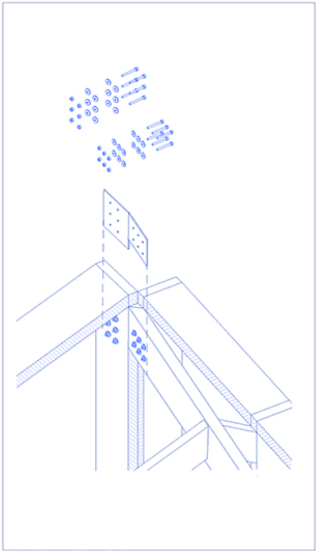
Union Viga - Pilar - Soleras
