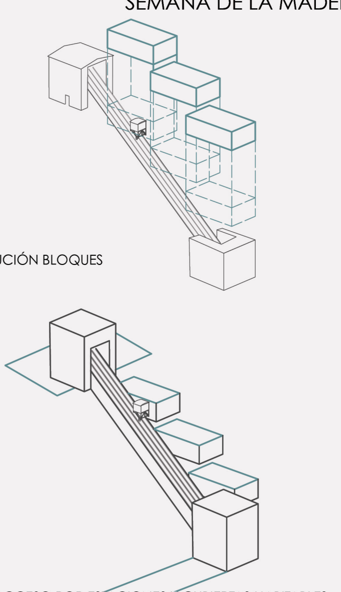
SEMANA DE LA MADERA DISTRIBUCIÓN BLOQUES PLAZAS ACCESO POR ESTACIONES Y CUBIERTAS HABITABLES
