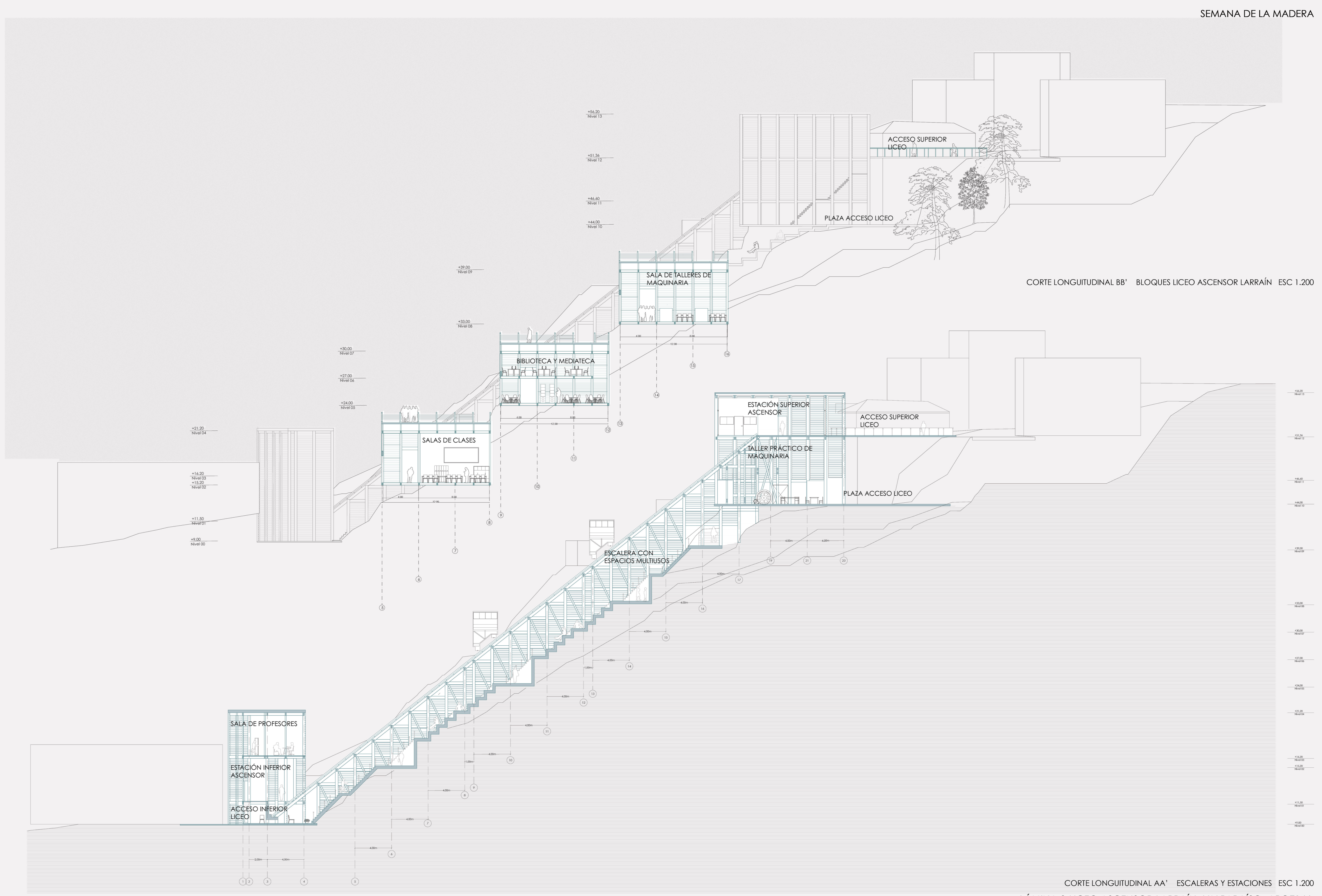
TALLER PRÁCTICO DE MANTENIMIENTO ELECTROMECÁNICO EN LA ESTACIÓN SUPERIOR DEL ASCENSOR
