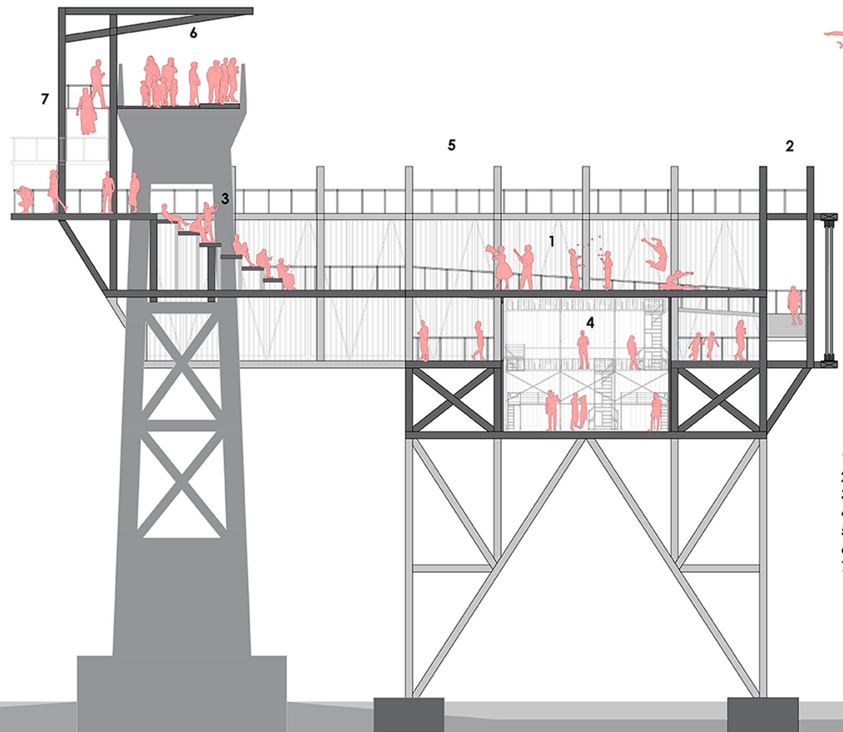
CORTE LONGITUDINAL A-A' 1:100
