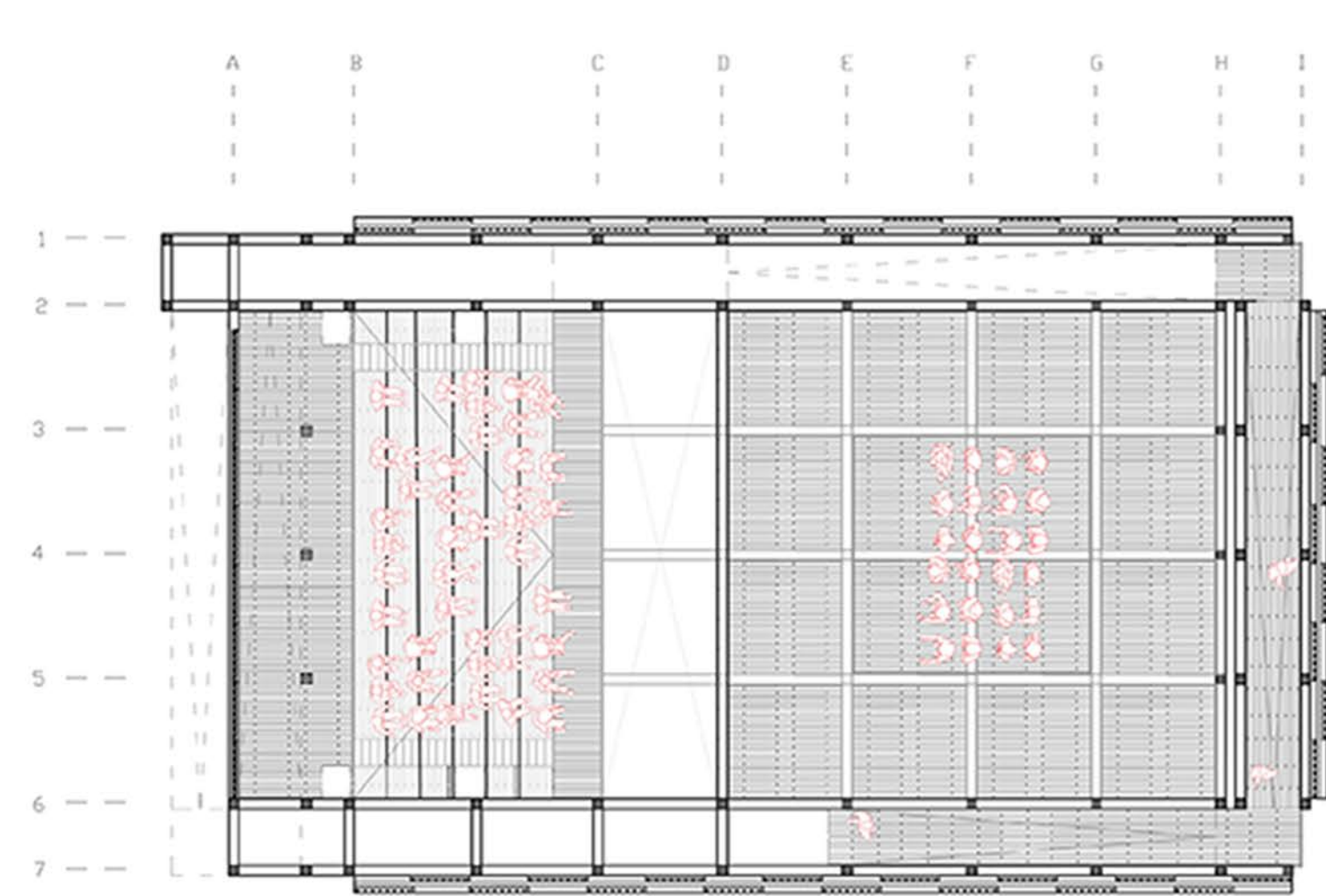
NIVEL ESCENARIO 1:200
