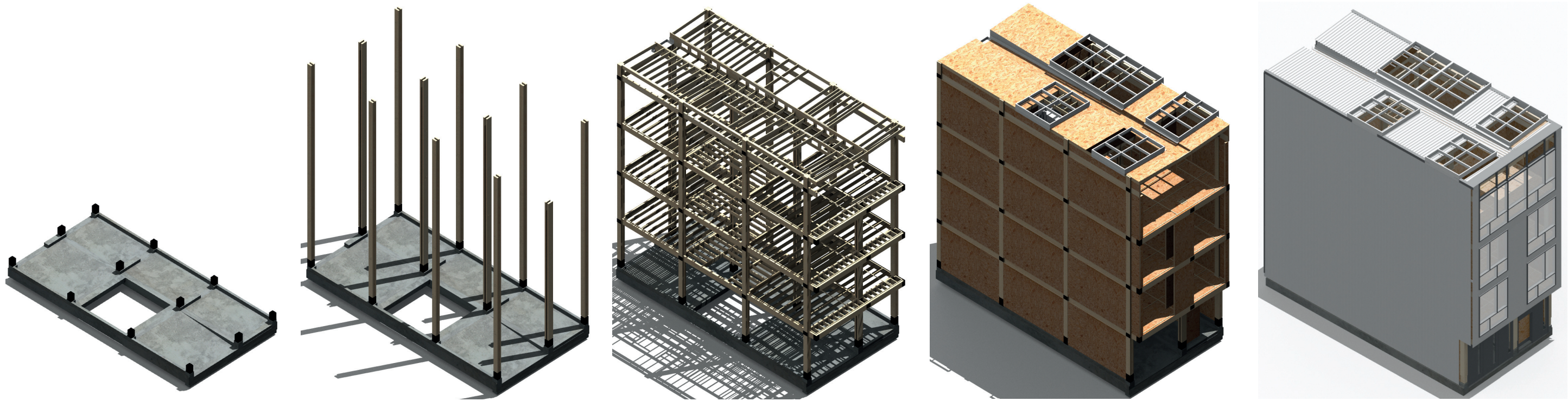
SECUENCIA CONSTRUCTIVA
