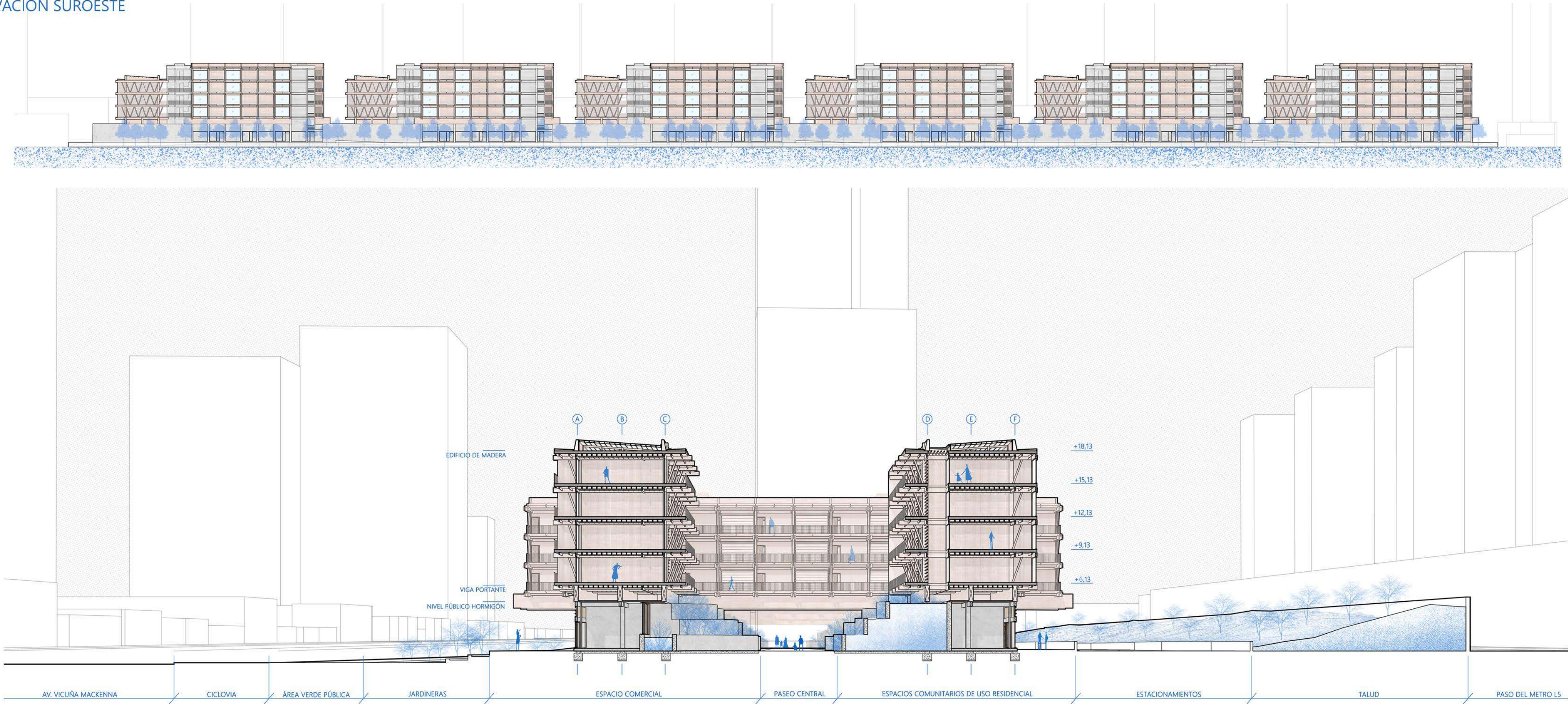
ELEVACIÓN SUROESTE
