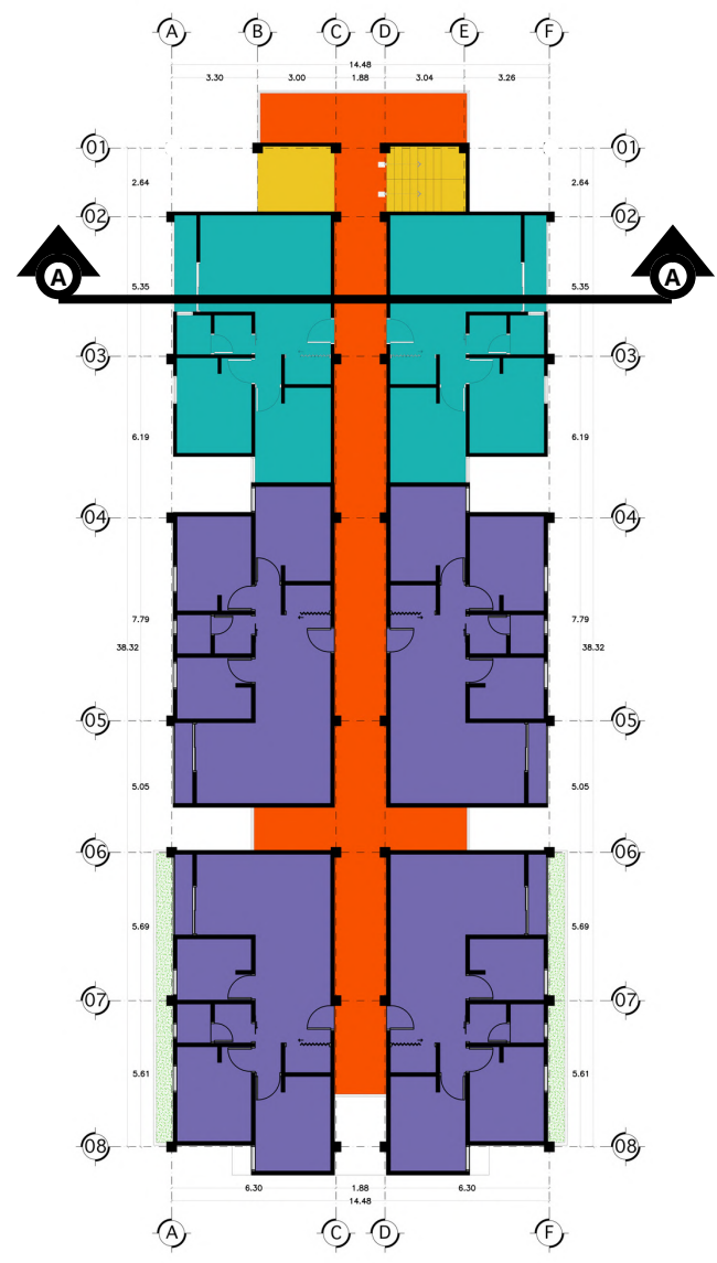
TORRE A - 2DO NIVEL
