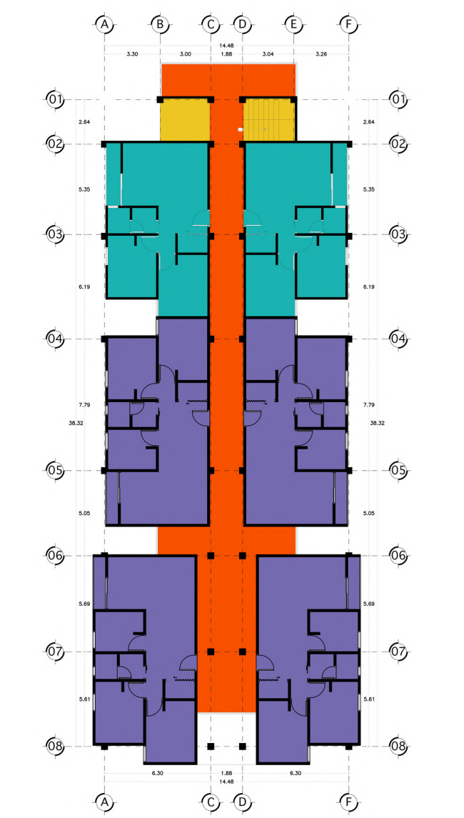
TORRE A - 3ER NIVEL
