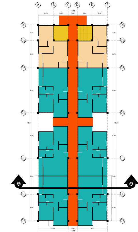
TORRE B - 1ER NIVEL
