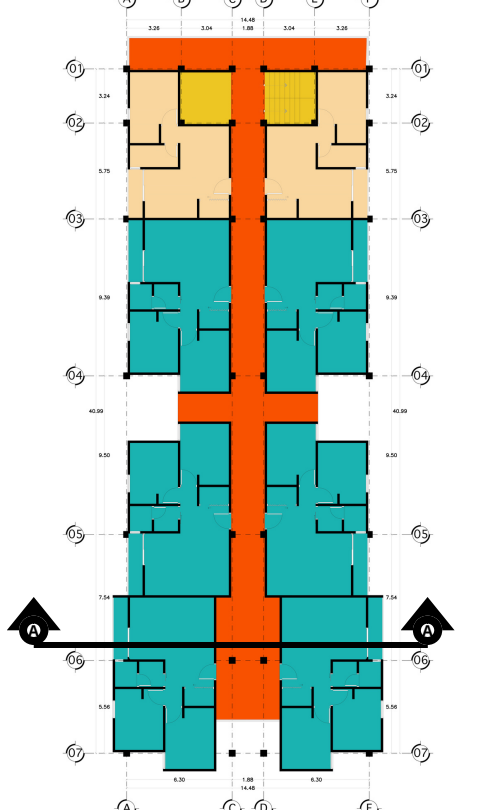
TORRE B - 2DO NIVEL
