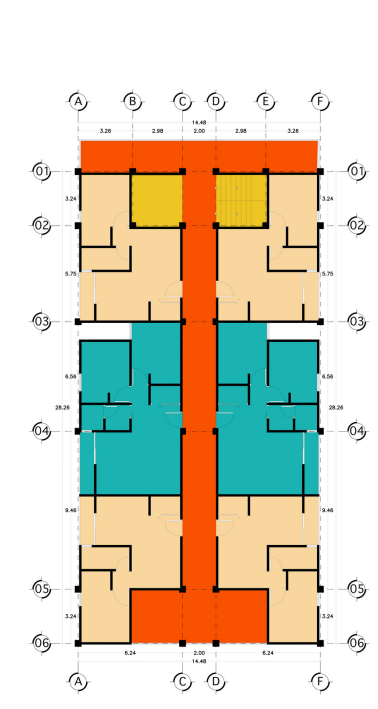
TORRE C - 1ER NIVEL
