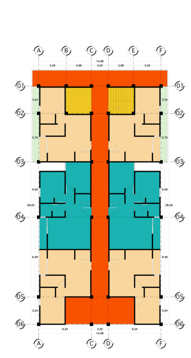
TORRE C - 2DO NIVEL
