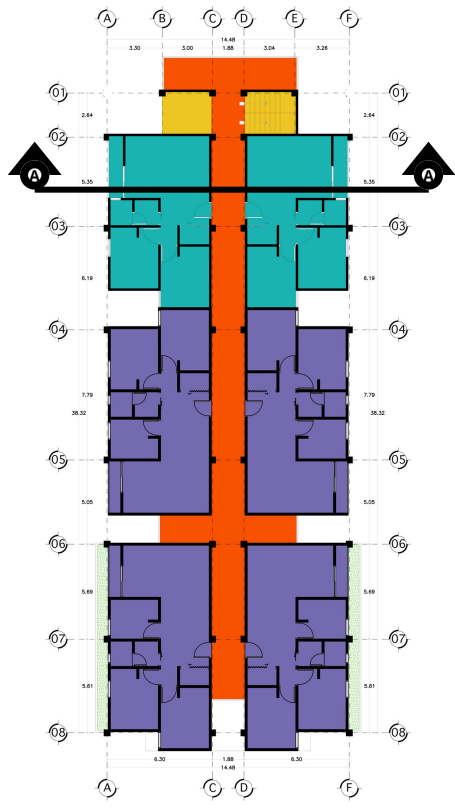
TORRE A - 2DO NIVEL
