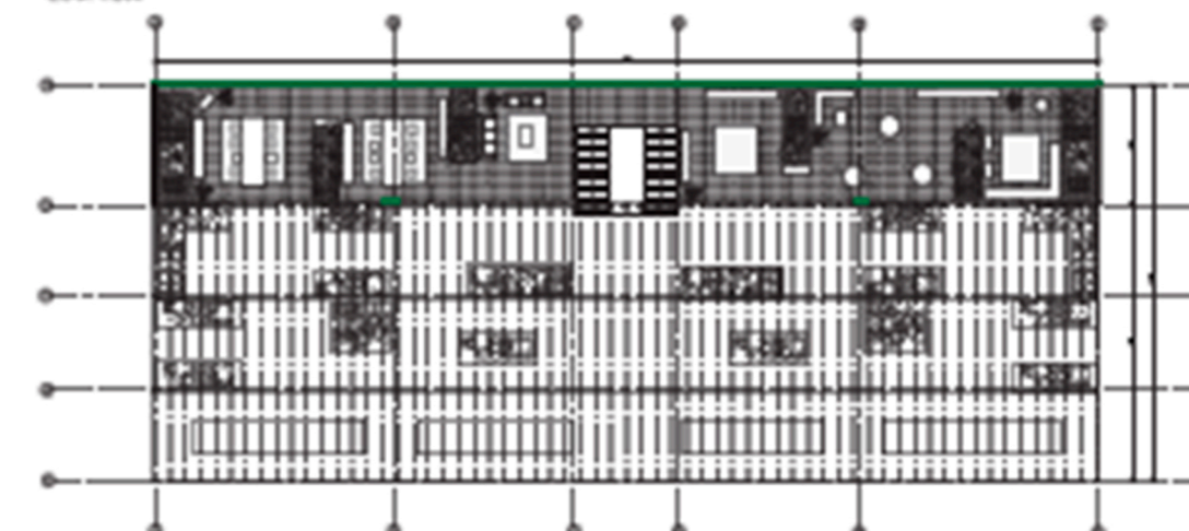
PLANTA CUARTO NIVEL EBC: 1:200
