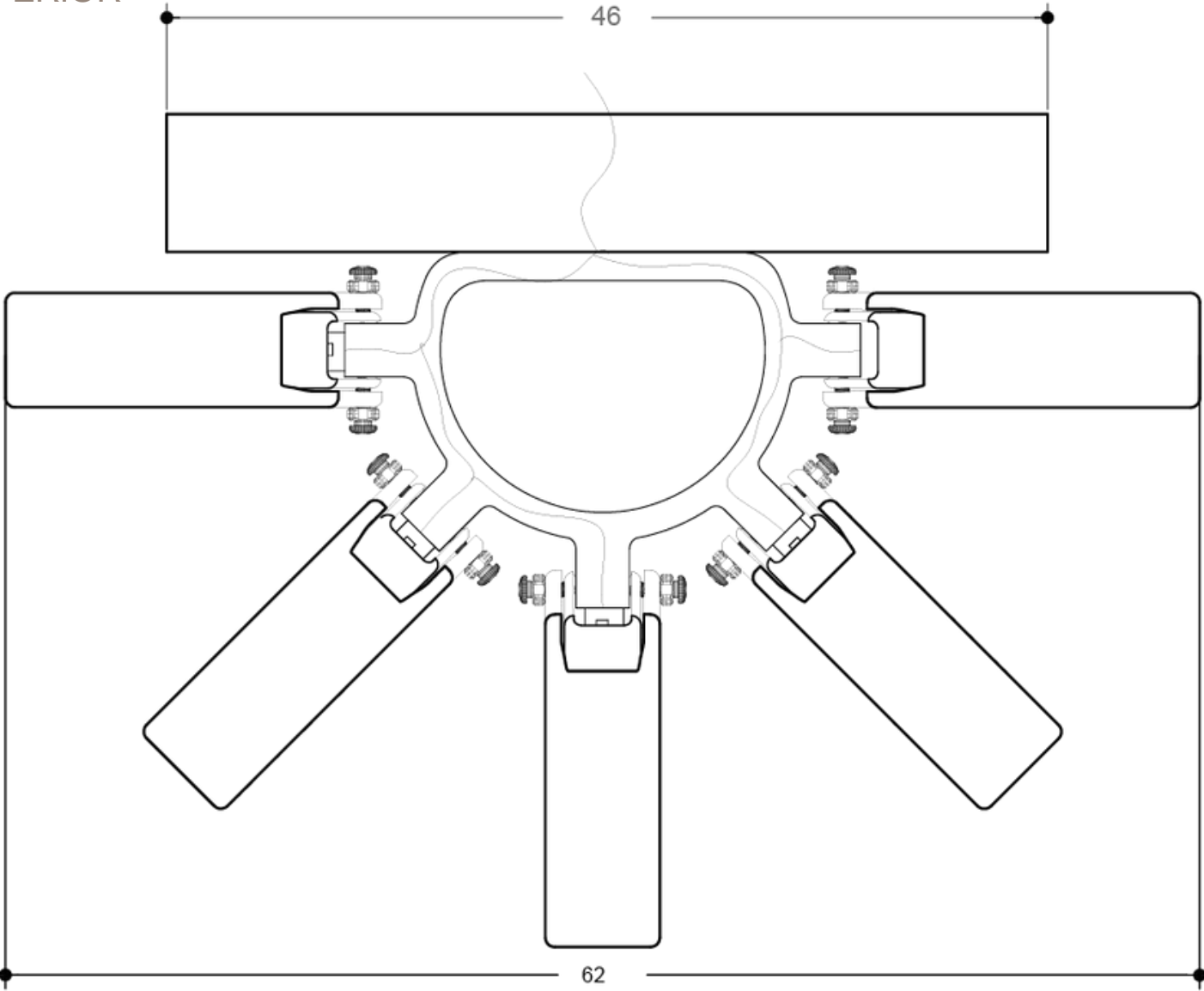
VISTA SUPERIOR
