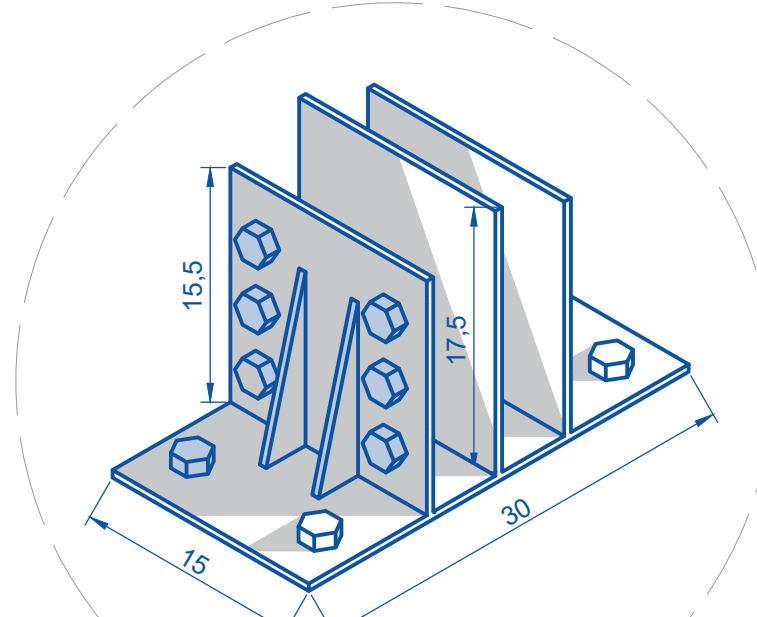
DET. B | HERRAJE VIGAS ESC 1:5
