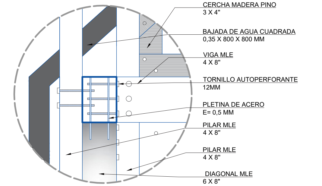
DET. 05 | UNIÓN PILAR - VIGA SUPERIOR
