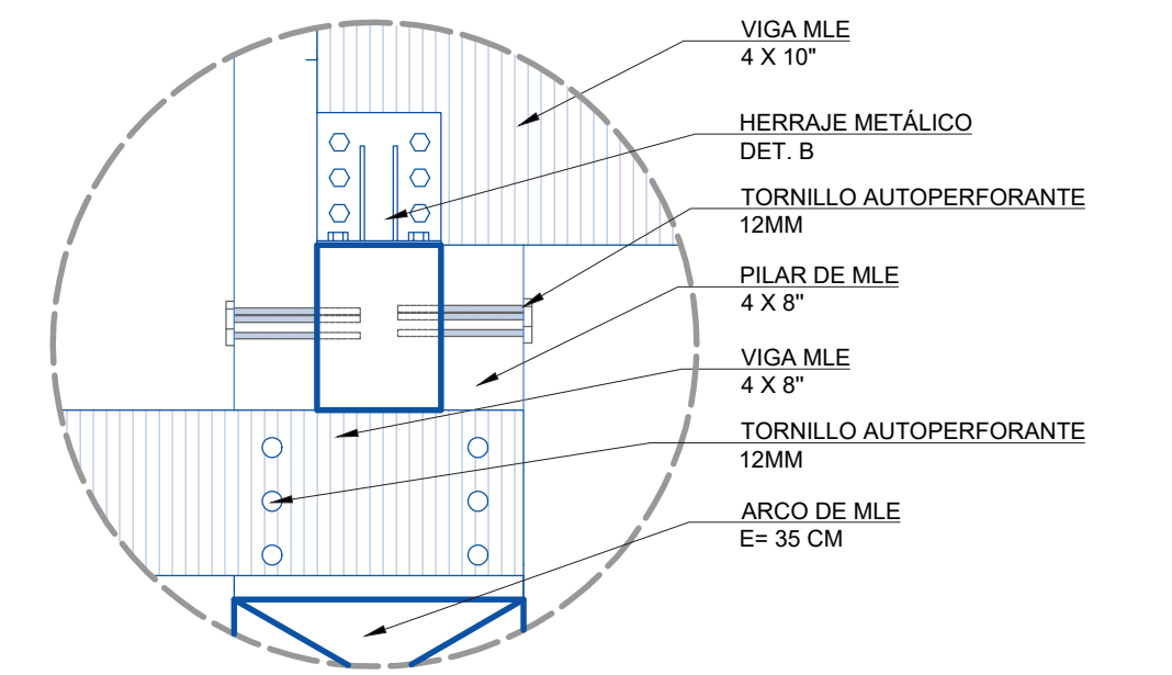
DET. 04 | UNIÓN PILAR - VIGAR INFERIOR
