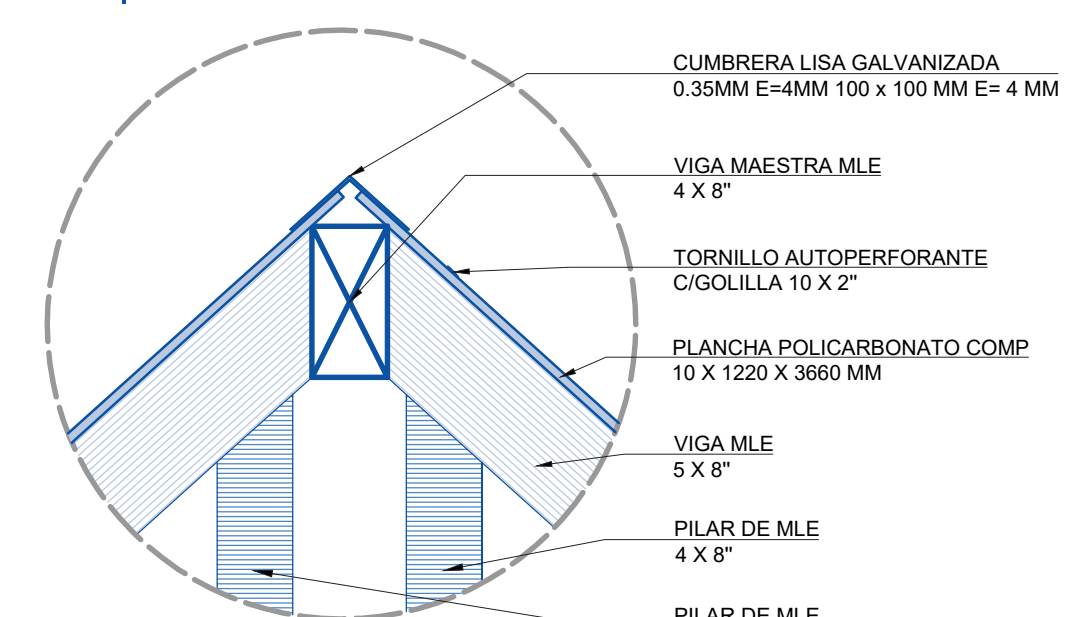
DET. 03 | CUMBRERA INVERNADERO
