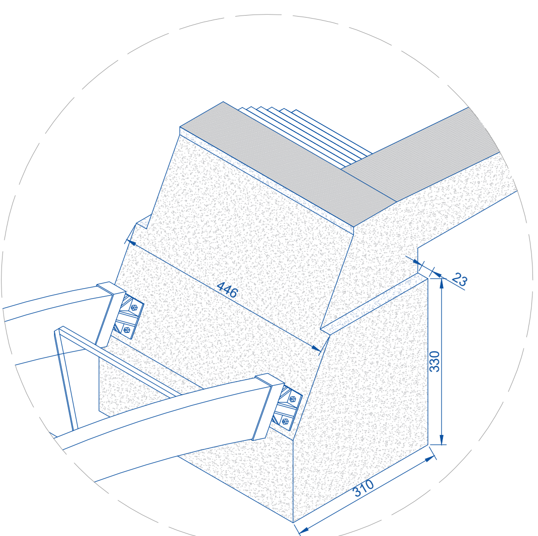
DET. D | FUNDACIONES ESC 1:75
