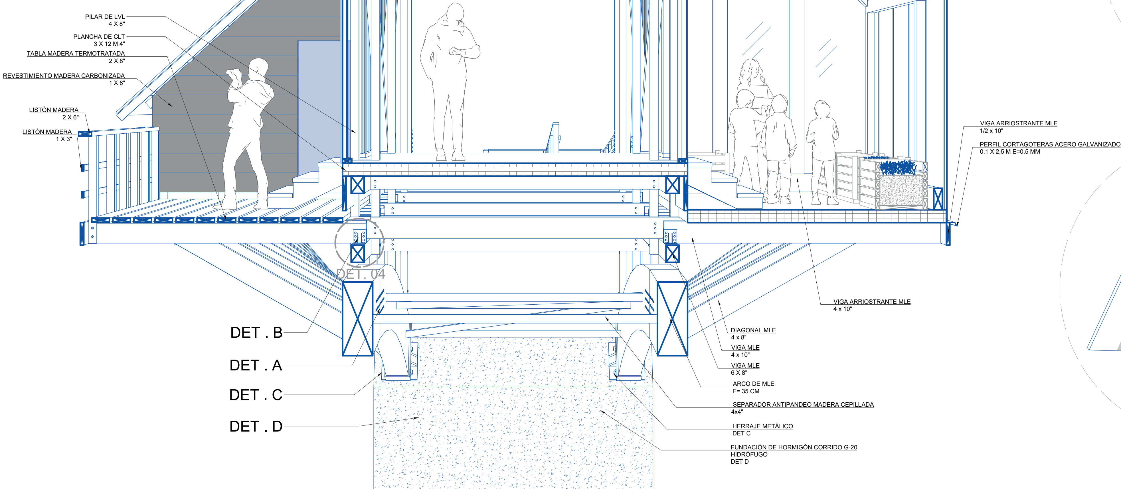
CORTE CONSTRUCTIVO FUGADO | ESC. 1:25
