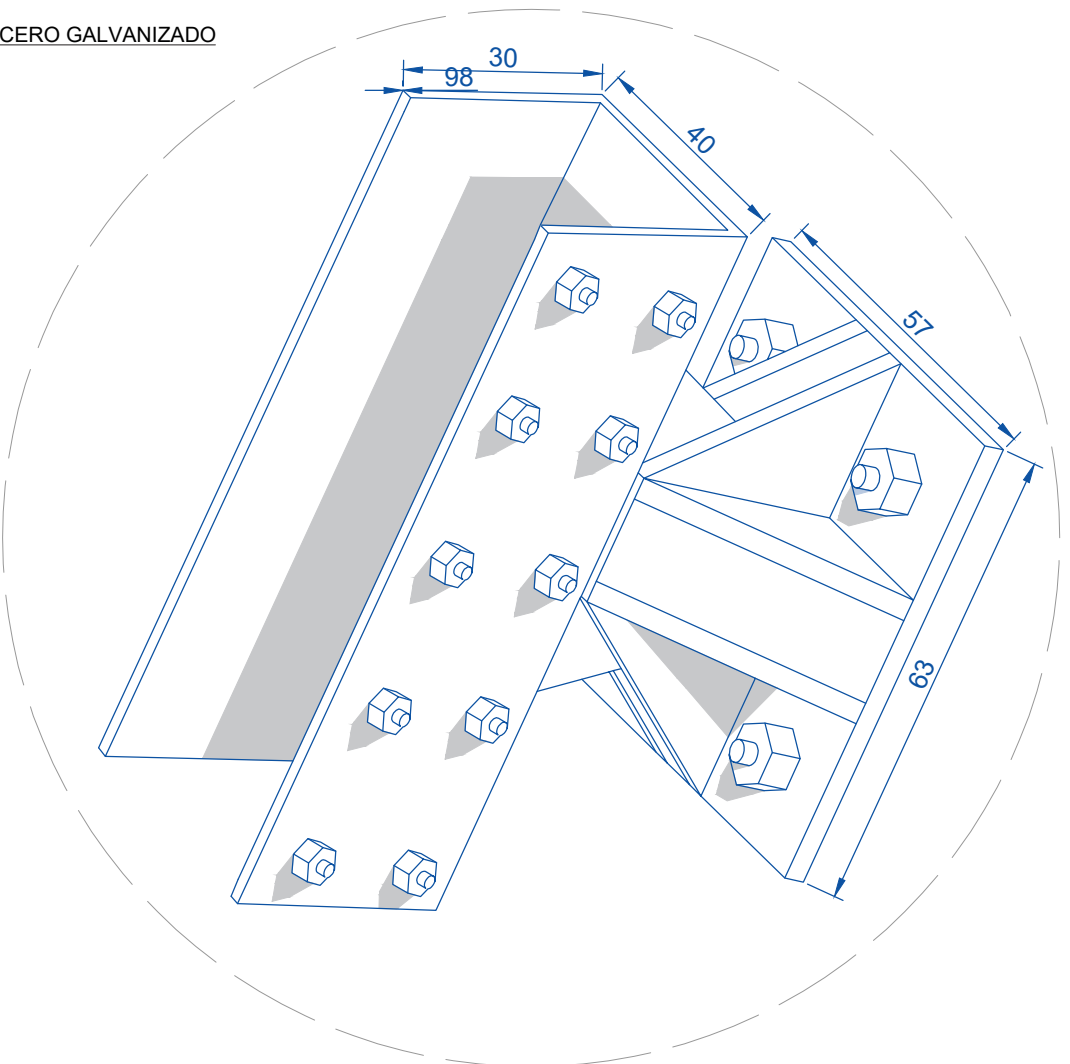
DET. C | HERRAJE ARCO - FUNDACIONES ESC 1:10
