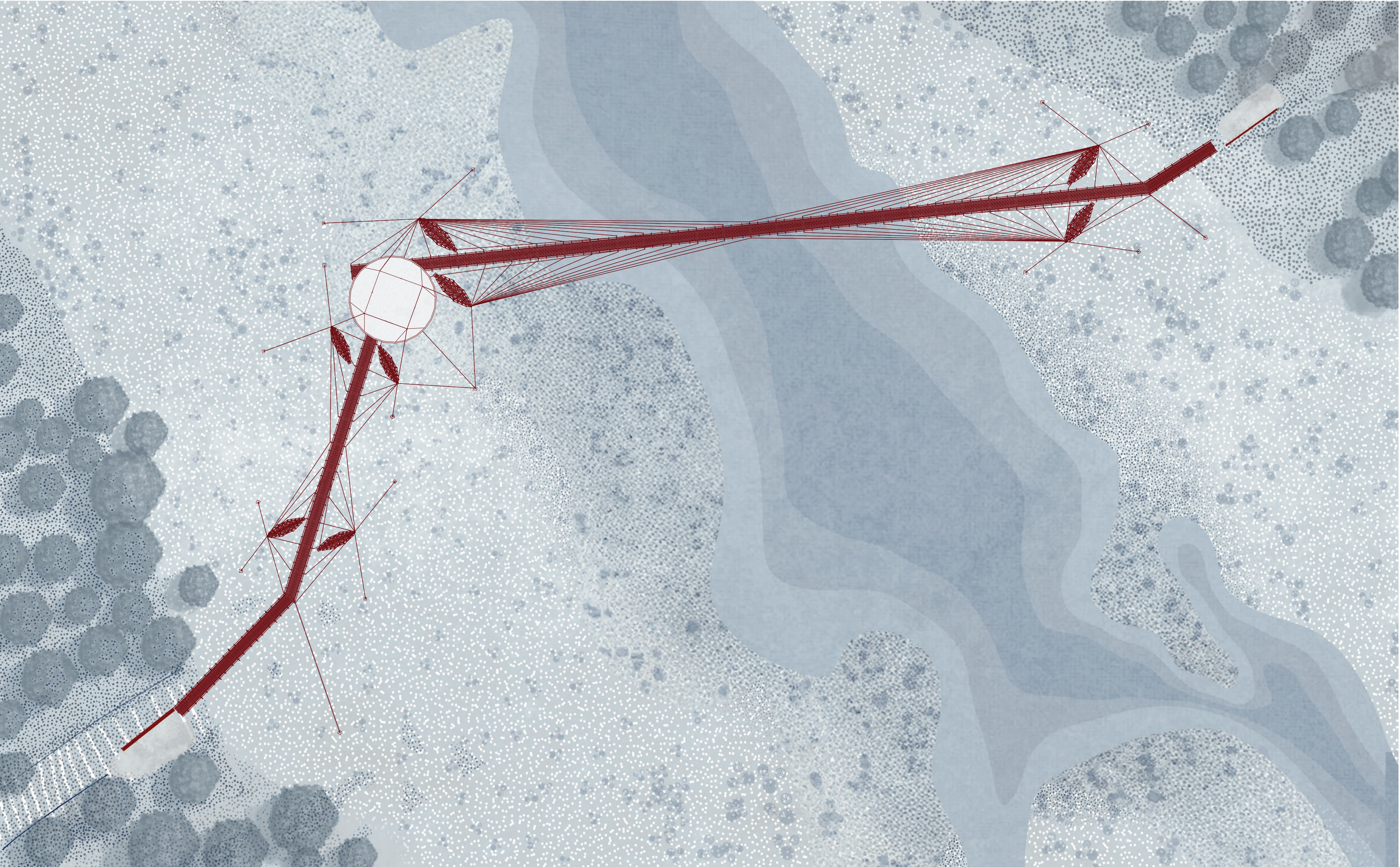
PLANTA PROYECTO ESC. 1:500
