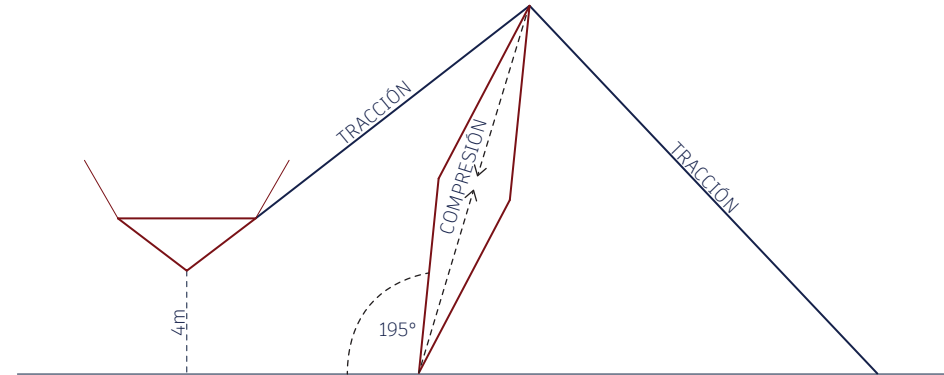
Descomposición Fuerzas
