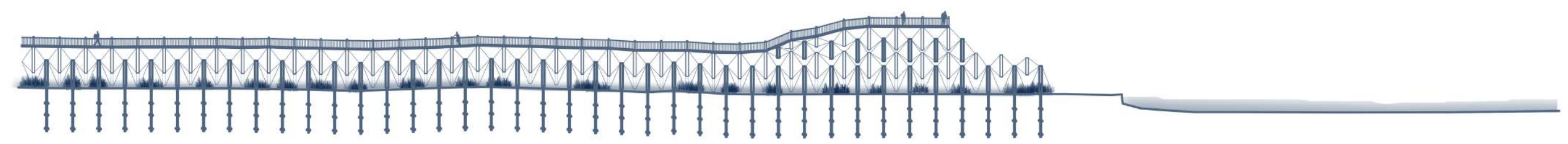
CORTE C-C'
