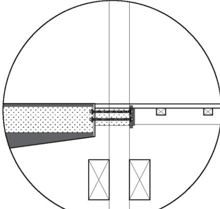
unión plataforma - puente
