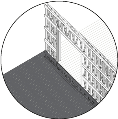
unión plataforma - puente
