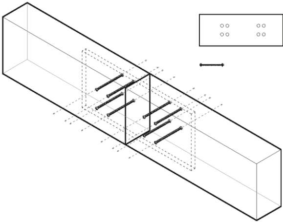
unión cable metálico - viga compuesta
