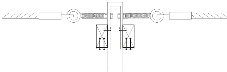
unión cable metálico - viga compuesta
