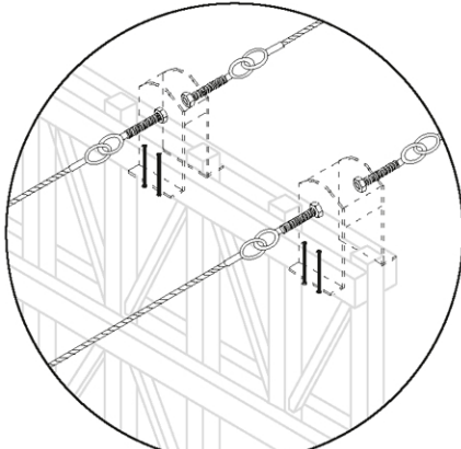
unión cable - viga
