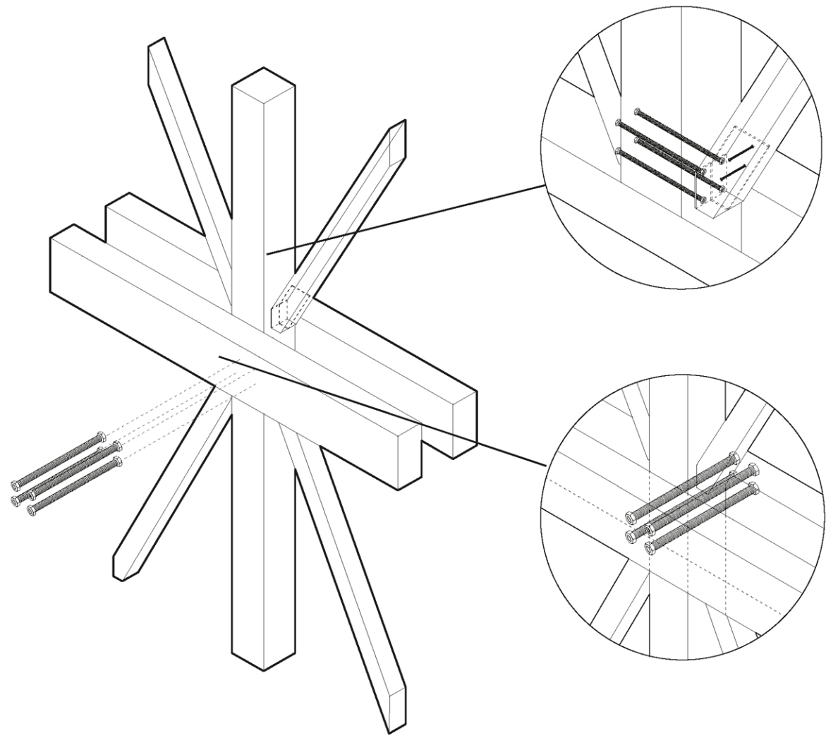
unión puntal - viga - diagonal
