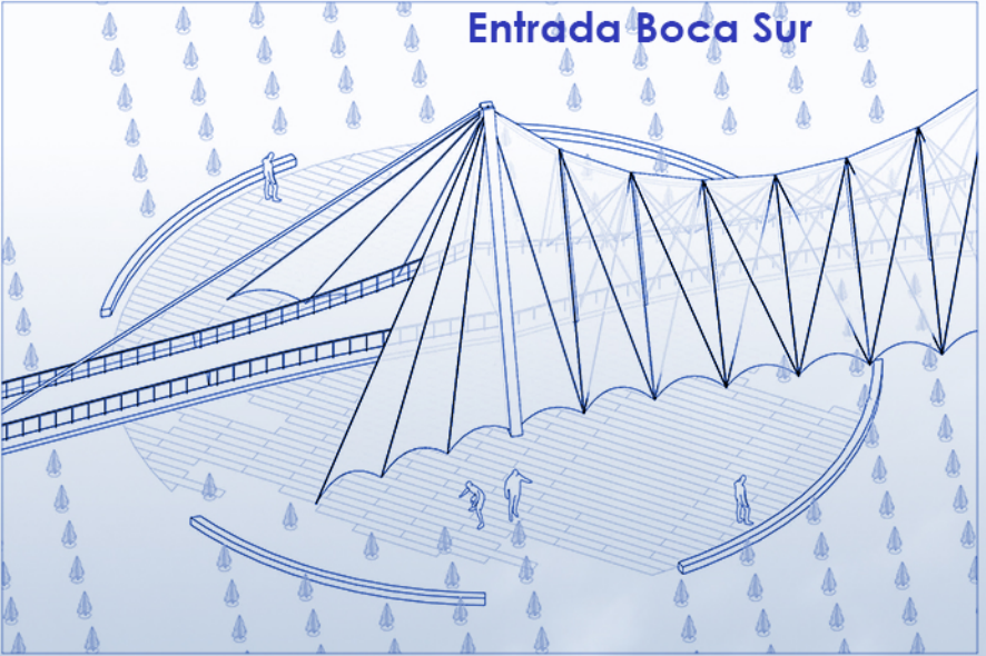
Axonométricas 1:150
