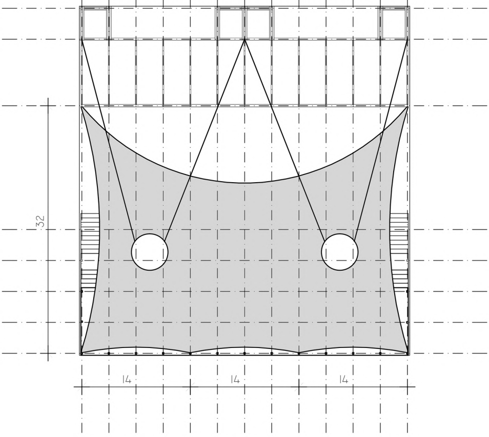
PLANTA CUBIERTA
