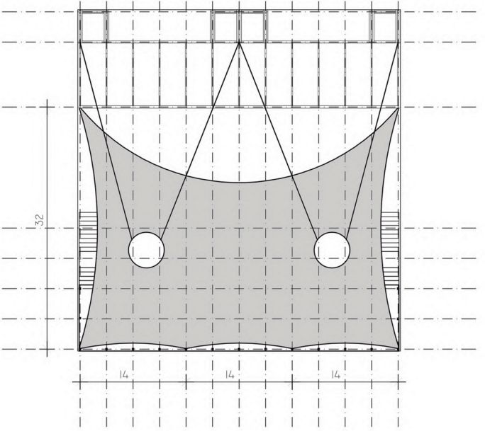
PLANTA CUBIERTA
