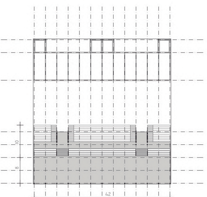
PLANTA SEGUNDO NIVEL
