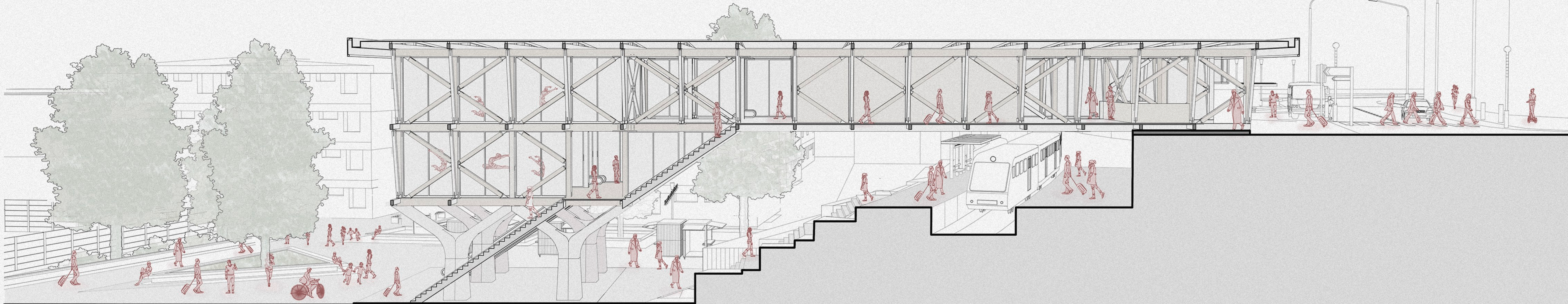
CORTE A-A'
