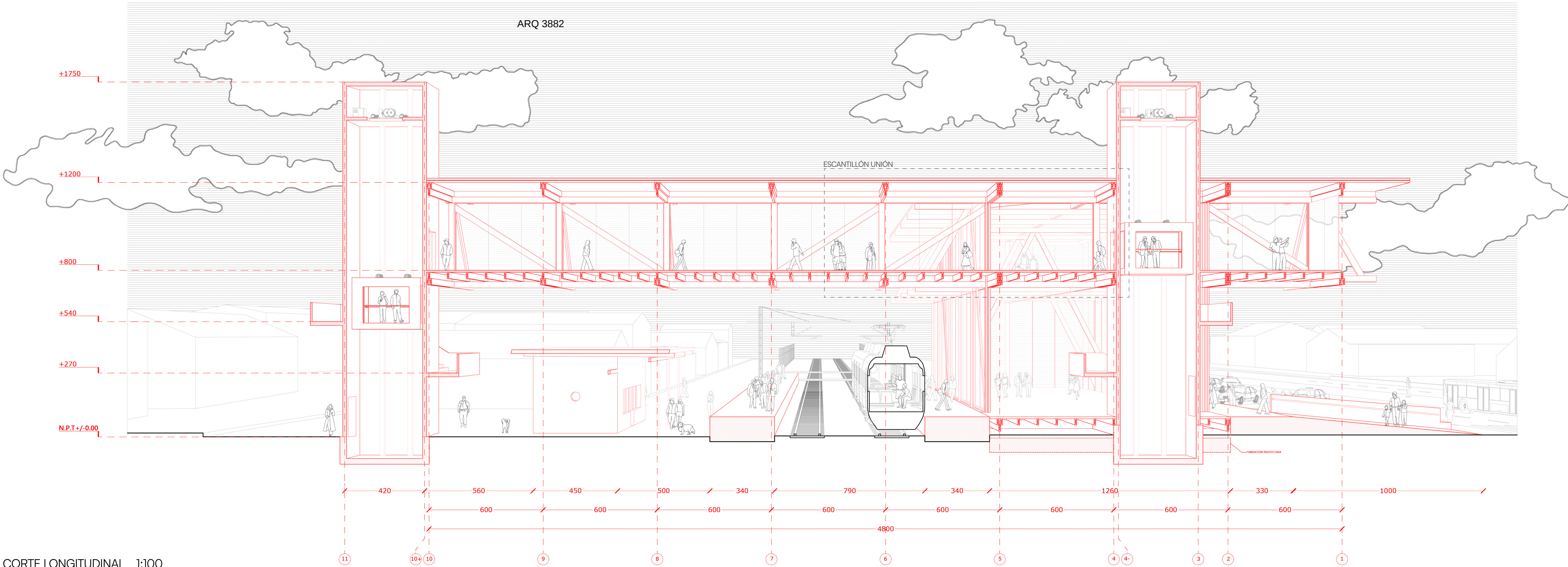
CORTE LONGITUDINAL 1:100
