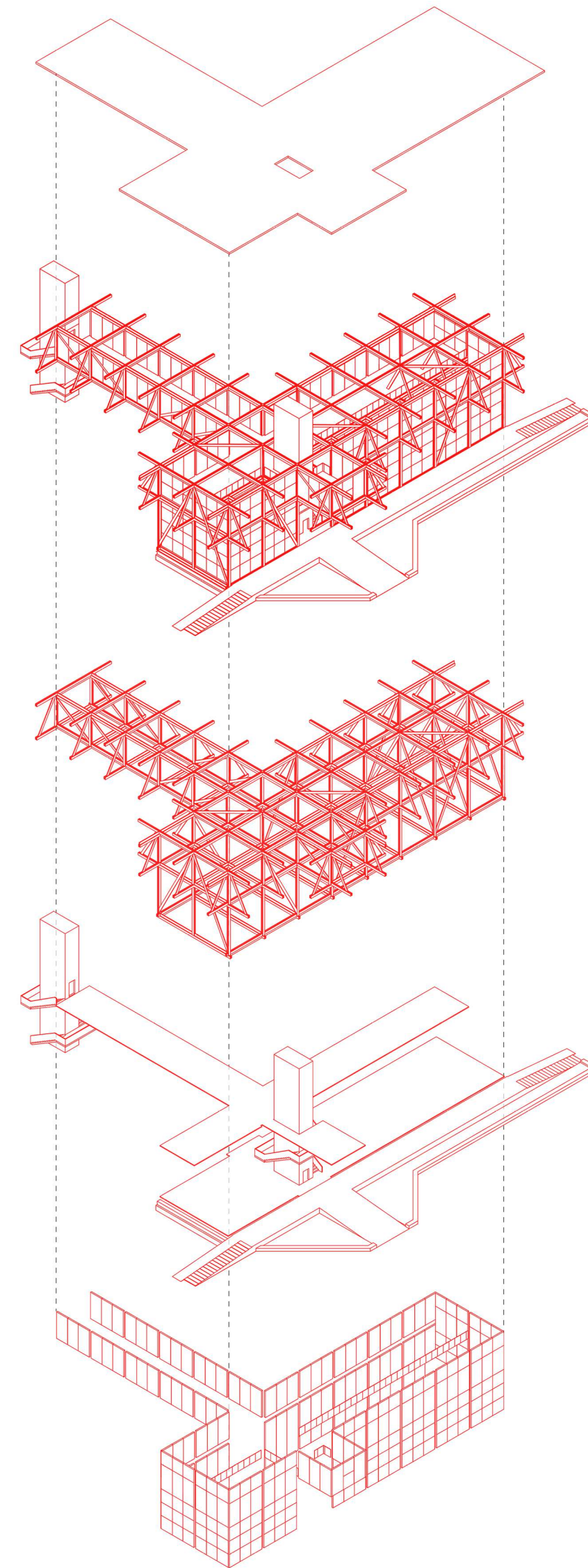
AXONOMÉTRICA ESPACIAL
