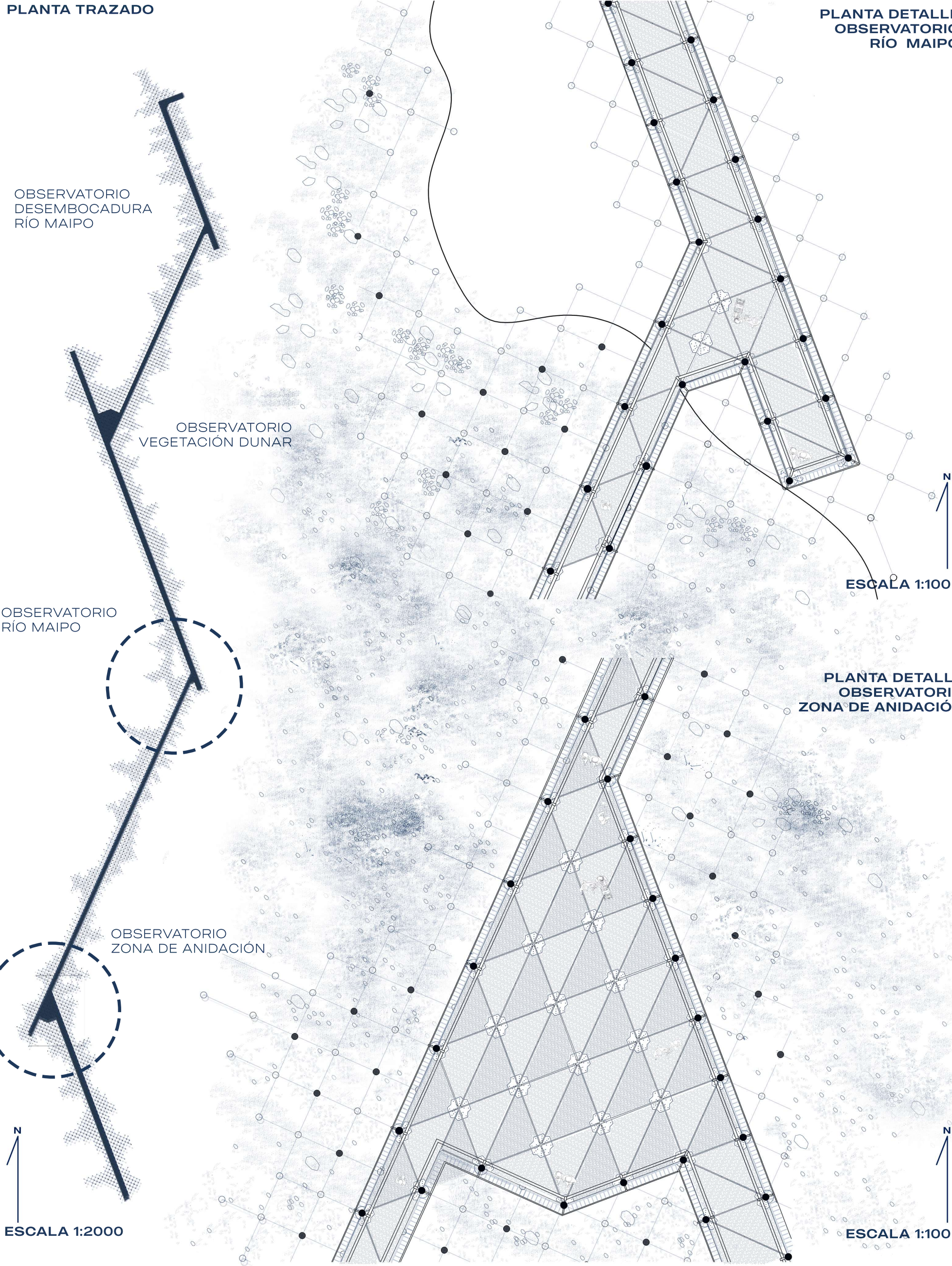
PLANTA TRAZADO
