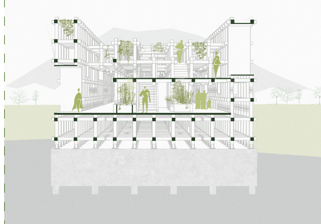
CORTE BB'
