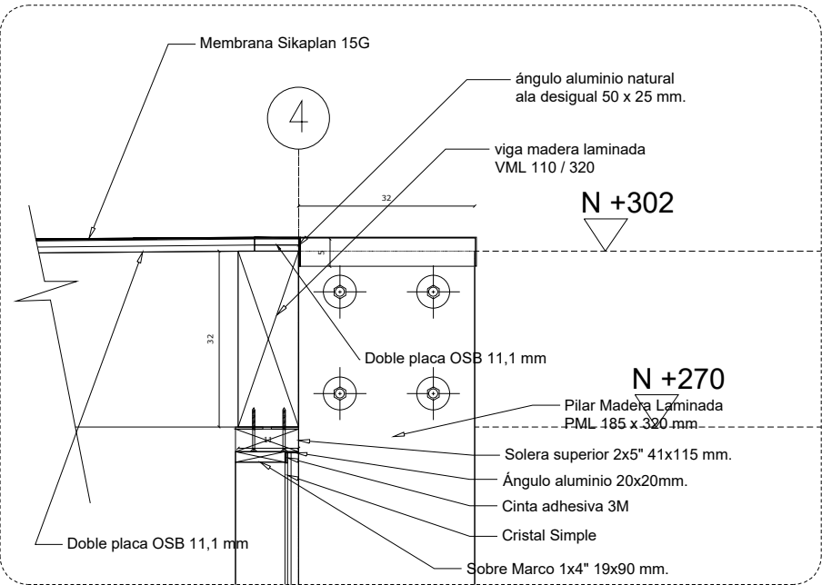
DET. 1 ESC. 1/10
