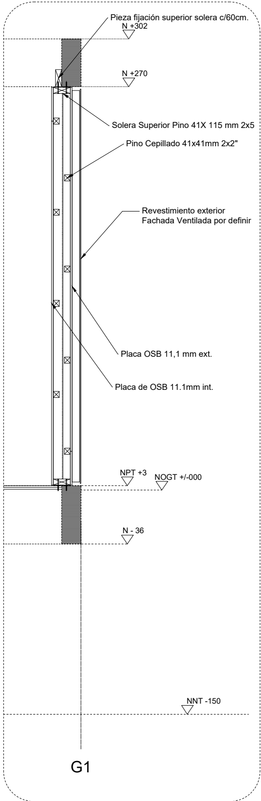
TABIQUE EXTERIOR ACÚSTICO DOBLE ESCANTILLÓN A ESC. 1/20
