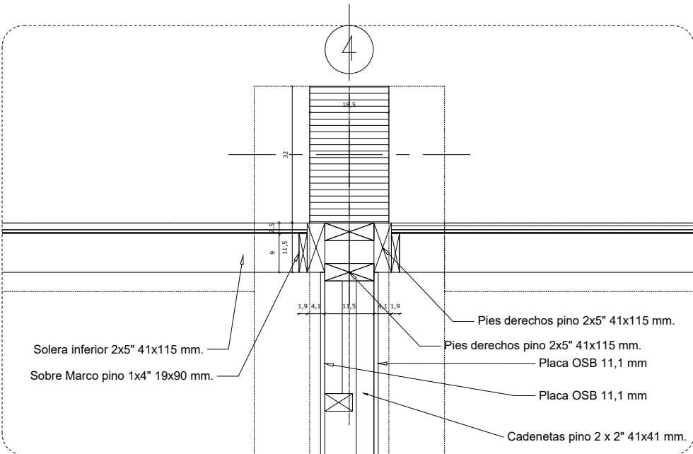
DET. 2 ESC. 1/10
