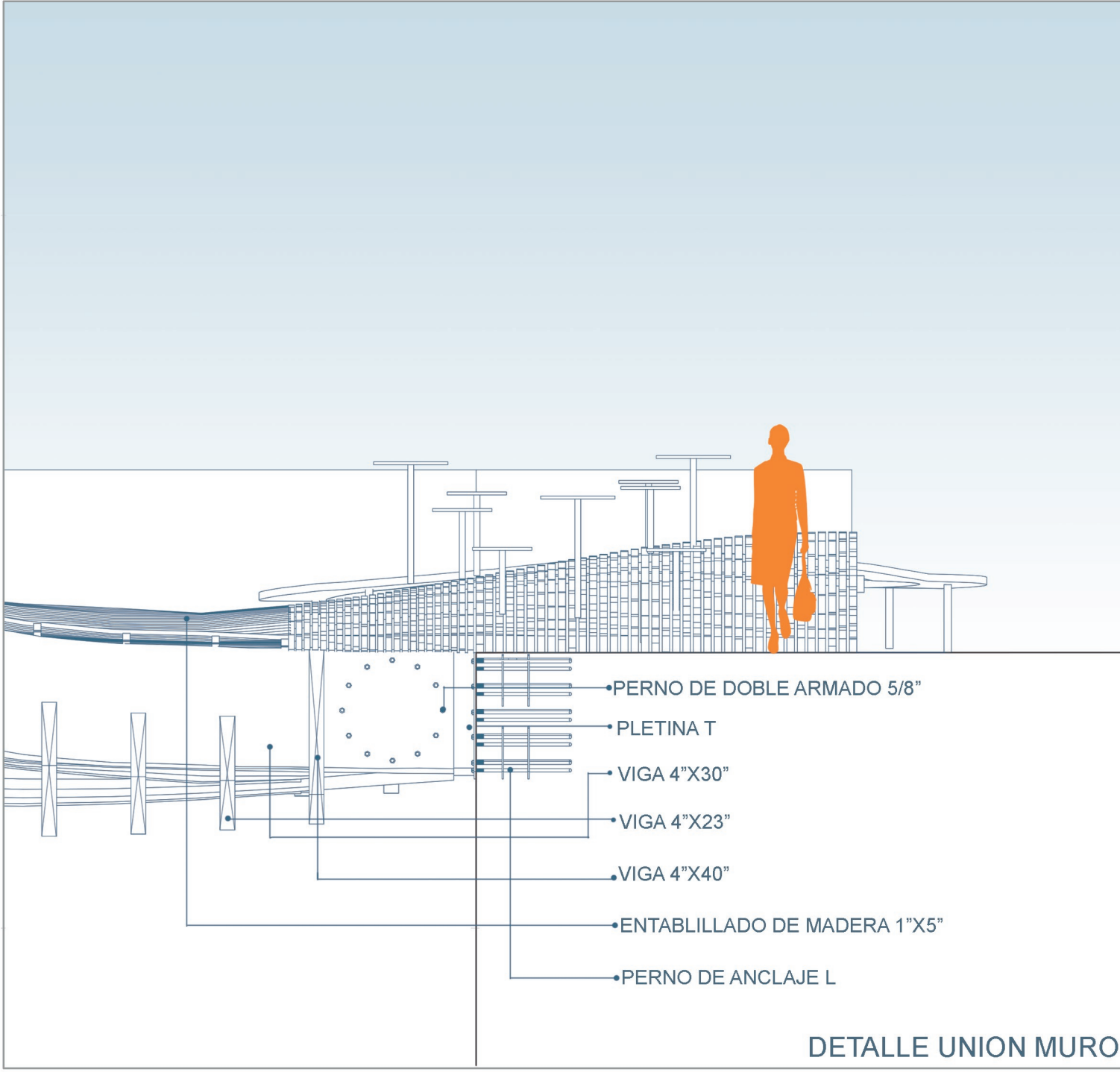
DETALLE UNION MURO LAMINA 2 ARQ3865
