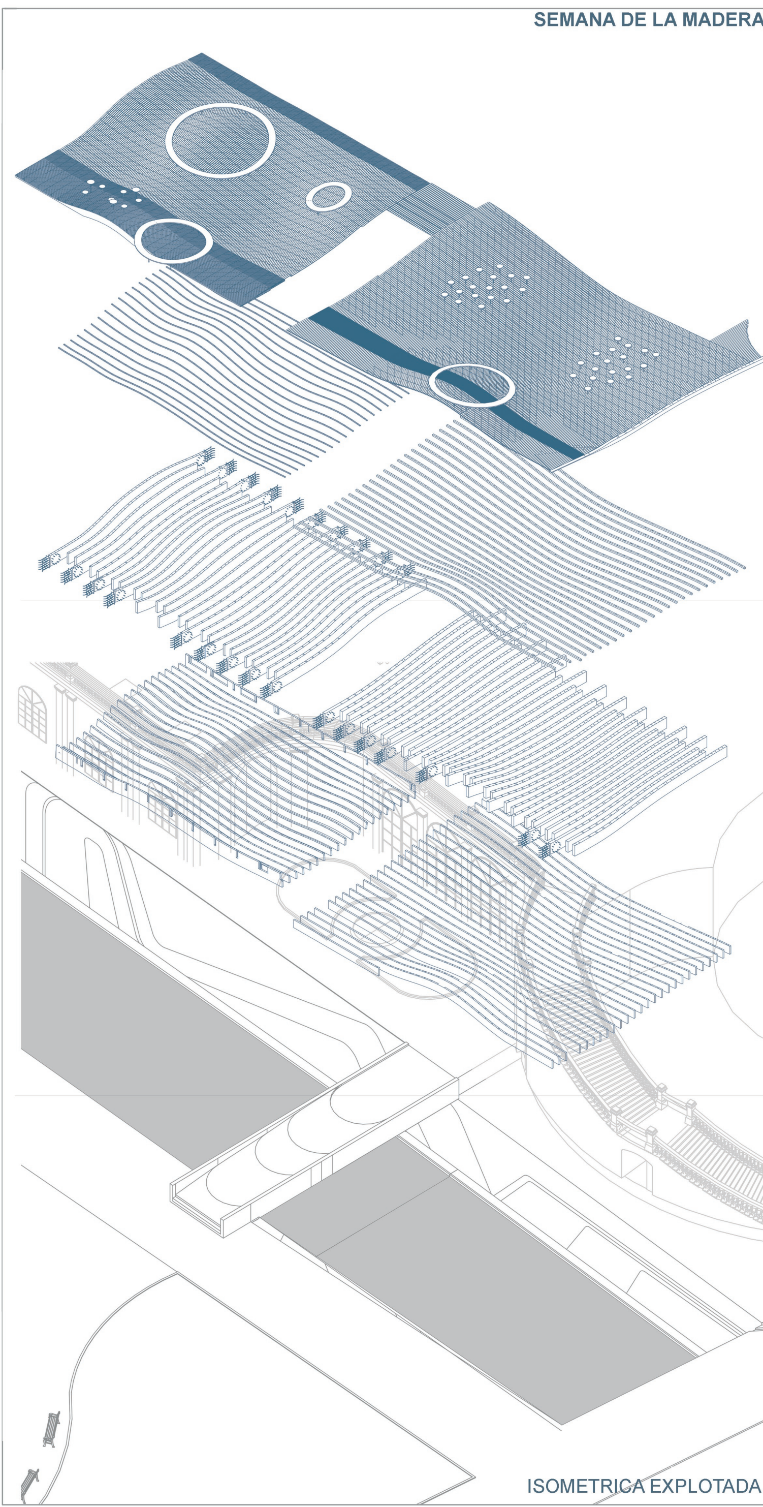
ISOMETRICA
