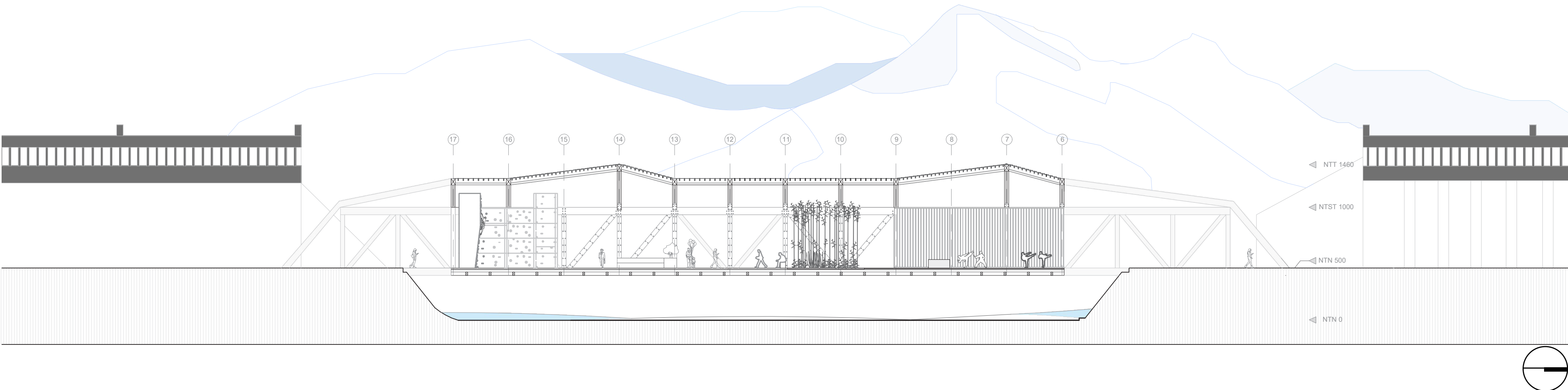
Corte Transversal 1/200
