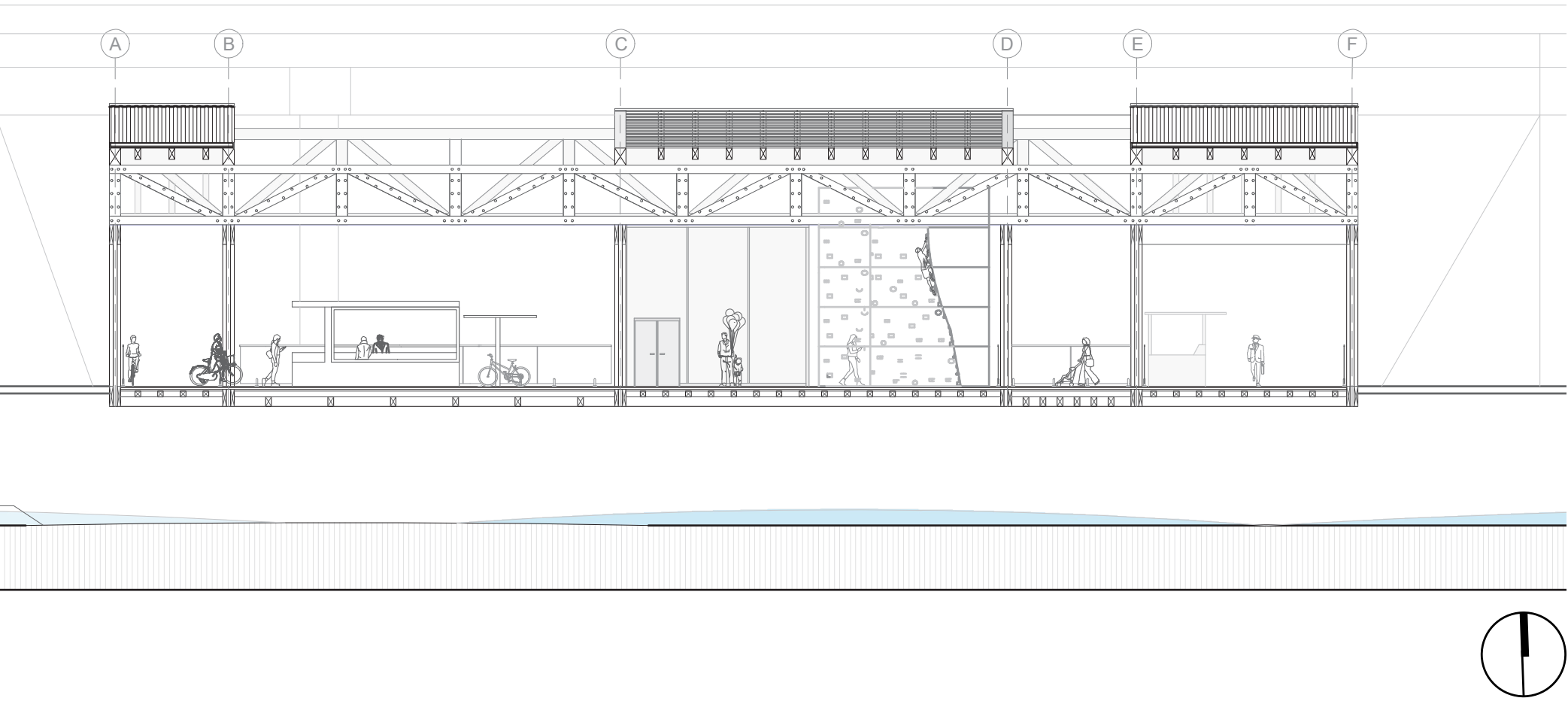
Corte Longitudinal 1/200
