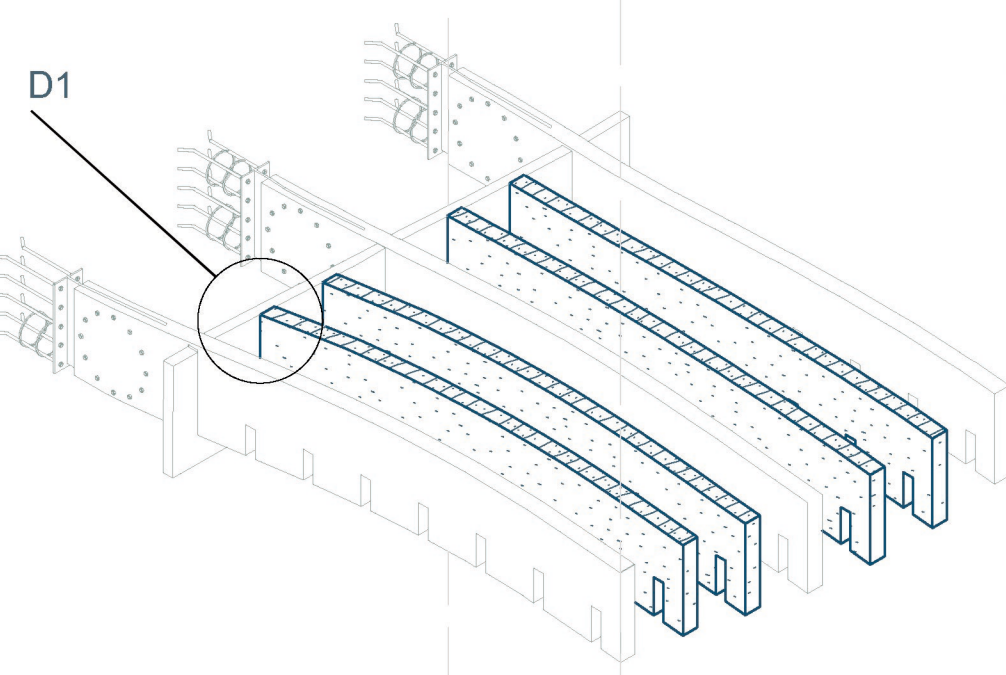
Instalación por herraje vigas secundarias a viga estructural B.
