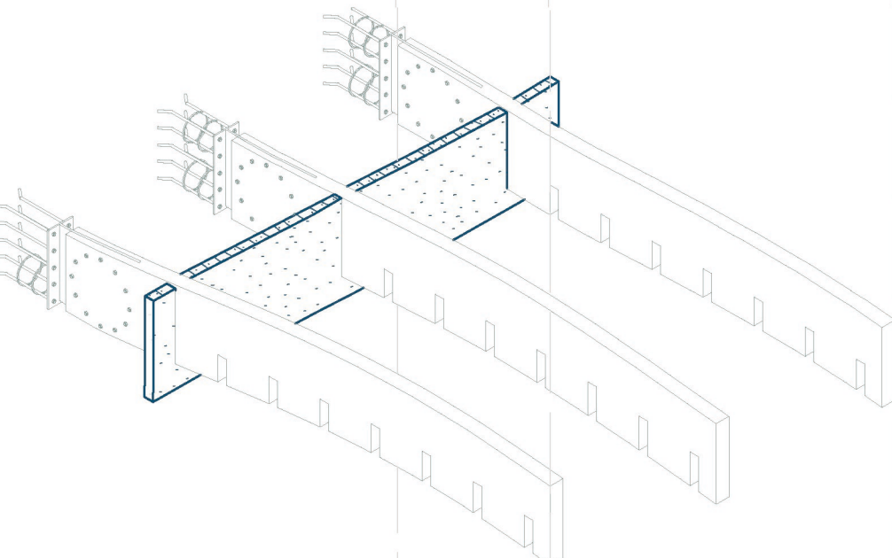
Instalación por ensamble - encaje viga estructural B
