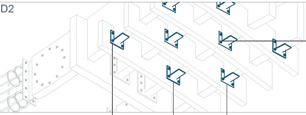
Instalación pletinas de acero "L" 5mm
