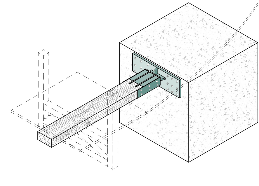
Uniones Puente a Talud
