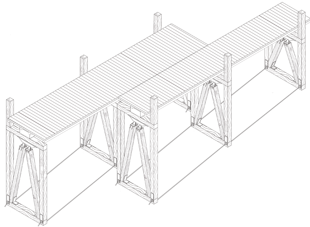
Axonometrica Puentes Desfasados
