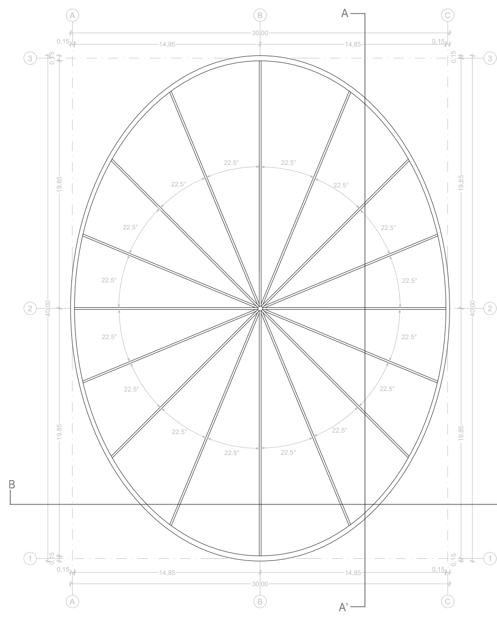
Planta pasarela Esc. 1 : 150
