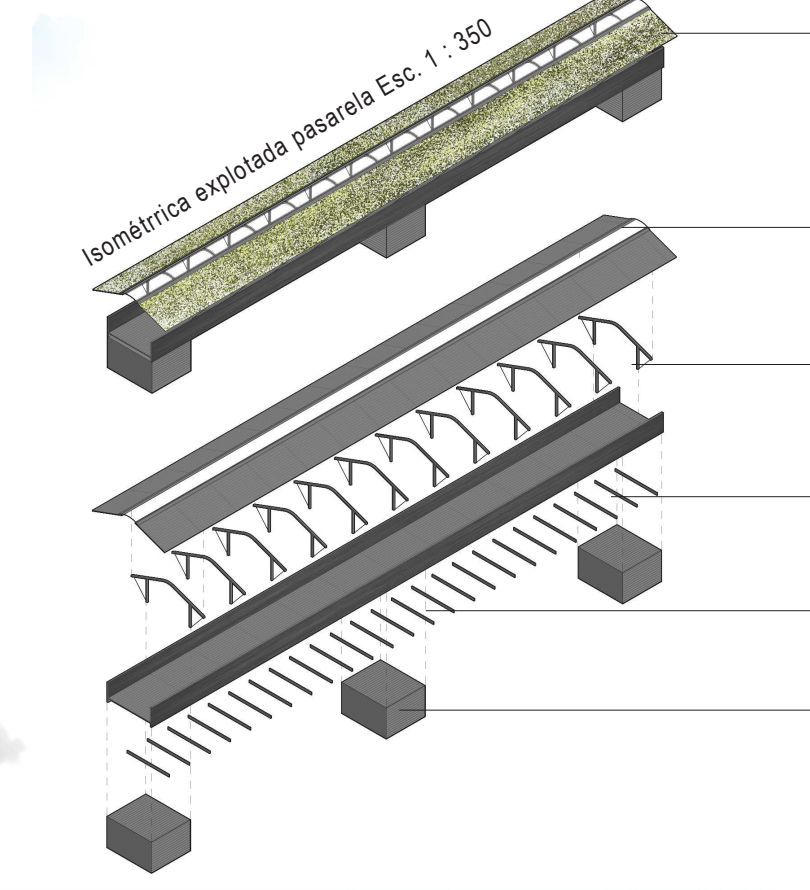
Pasarela techada 3.2 x 30 mts
