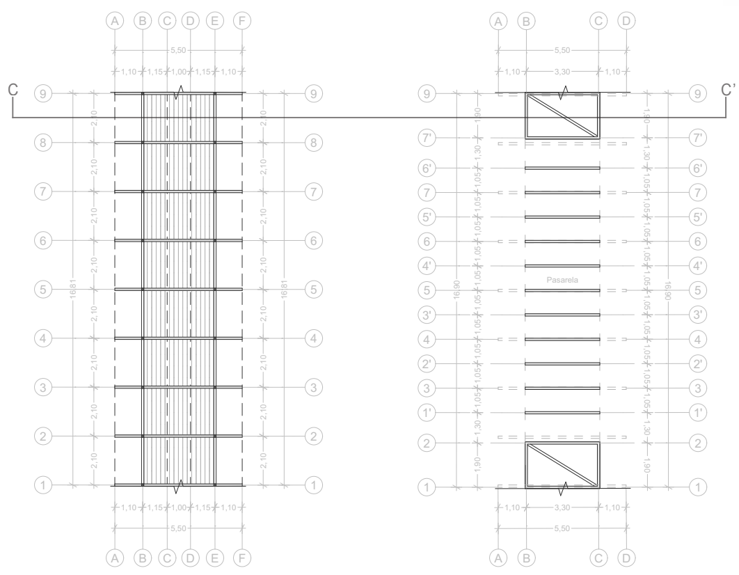
Planta pasarela Esc. 1 : 150
