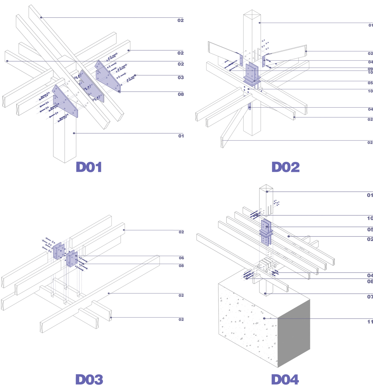
DETALLES CONSTRUCTIVOS
