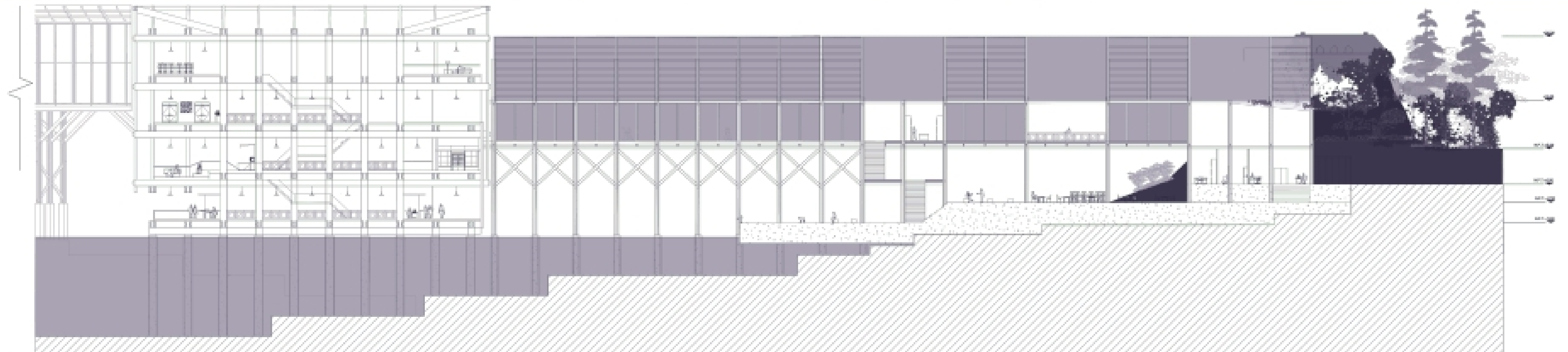
Corte B-B | Esc: 1/250
