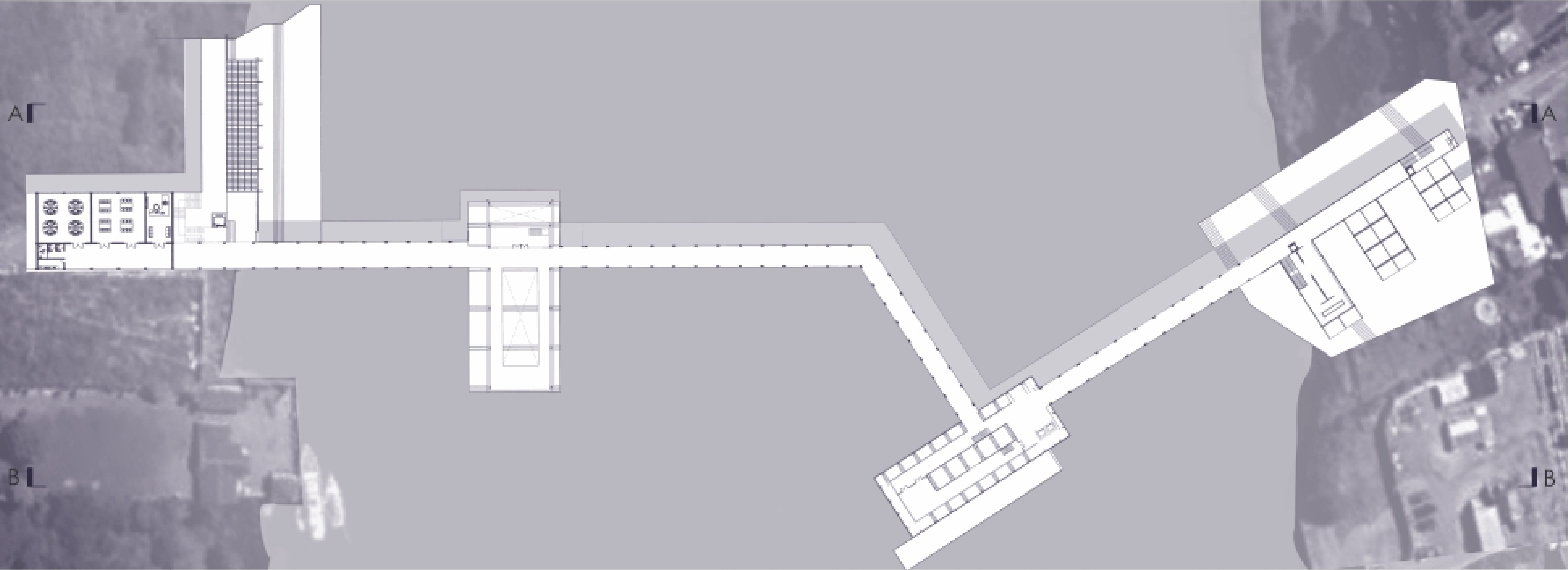
Planta General | Esc: 1/250
