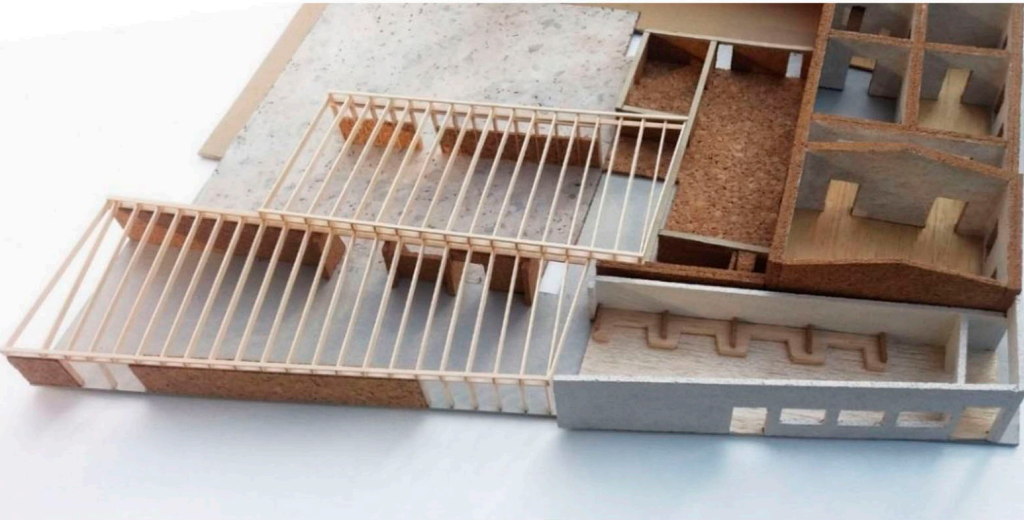
Envigado soportado por los centenarios muros de adobe. Emplazamiento en Zona Típica protegida.
