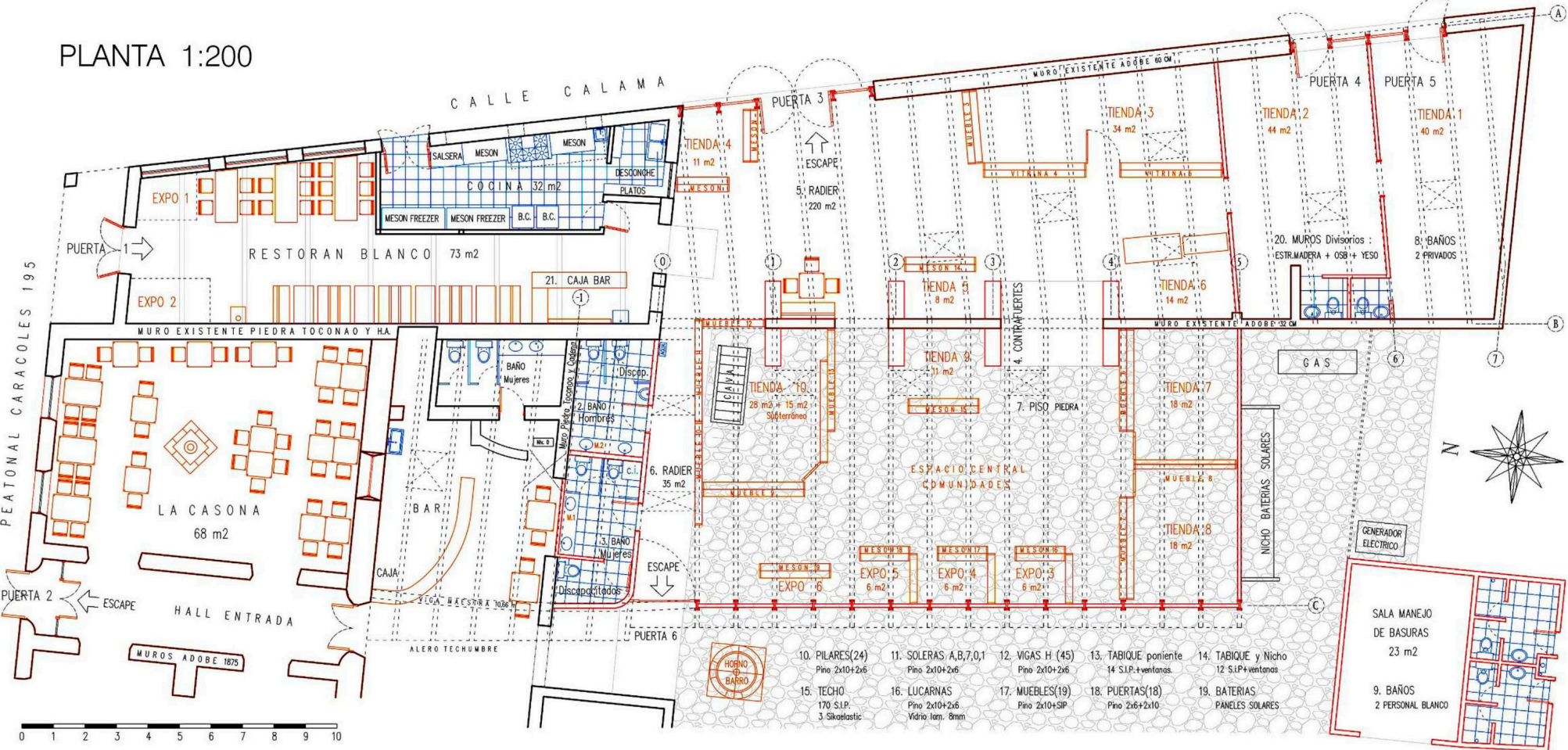
El sistema estructural de soleras, vigas y pilares parece volar sobre los pesados muros, y al mismo tiempo los confina y refuerza.
