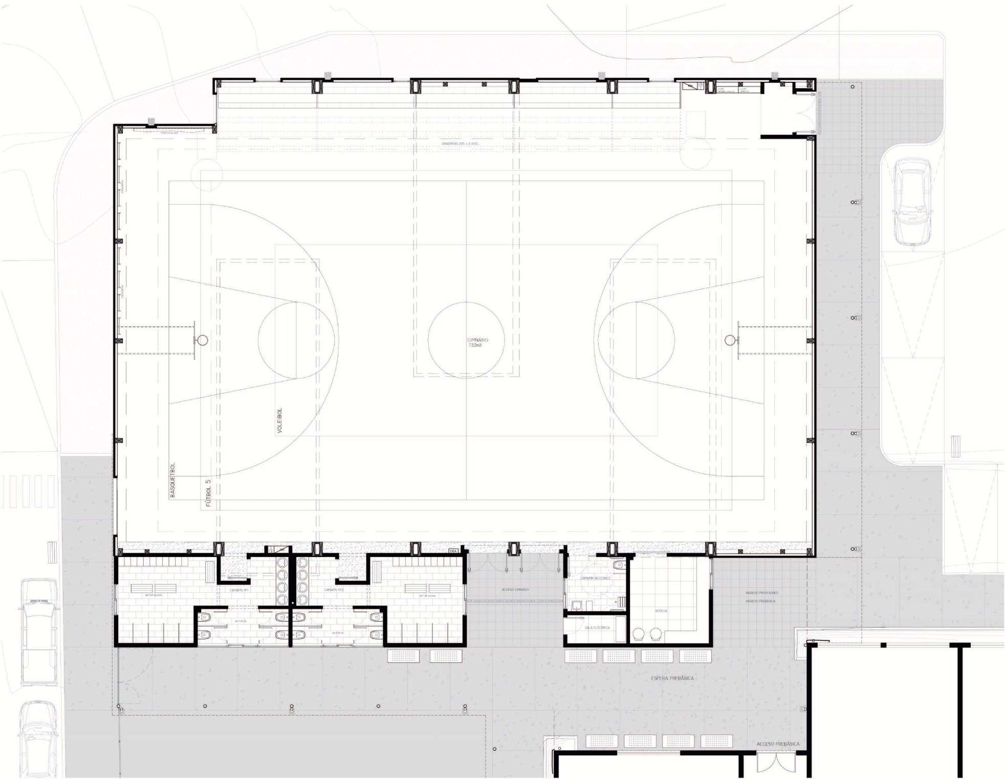
planta
