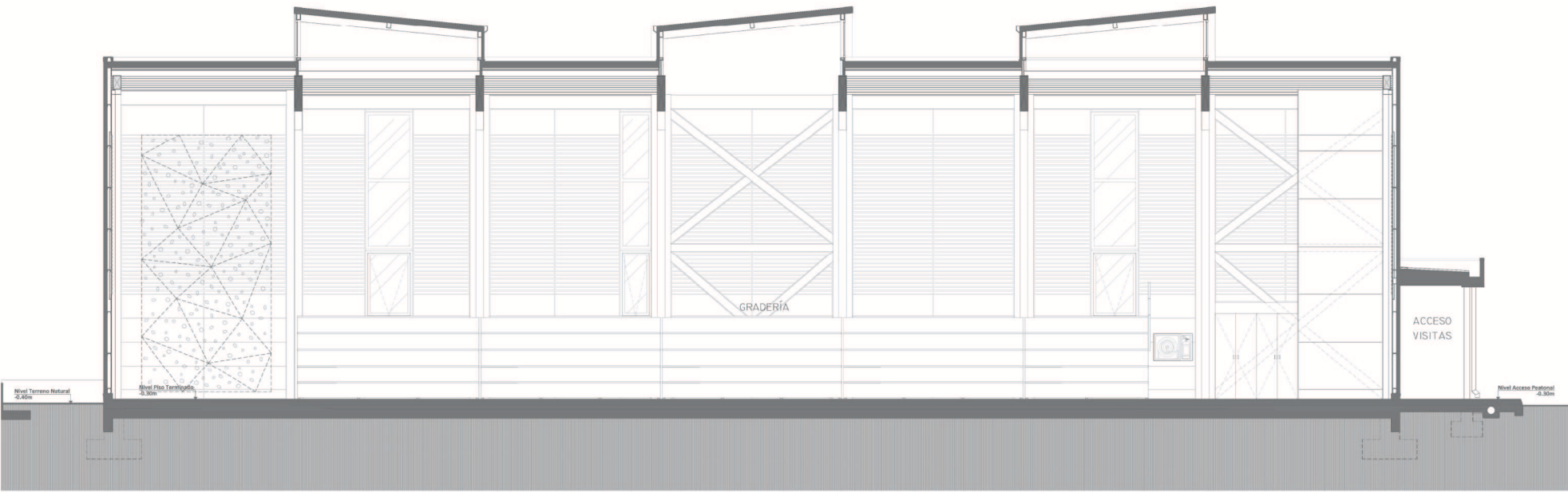
corte longitudinal
