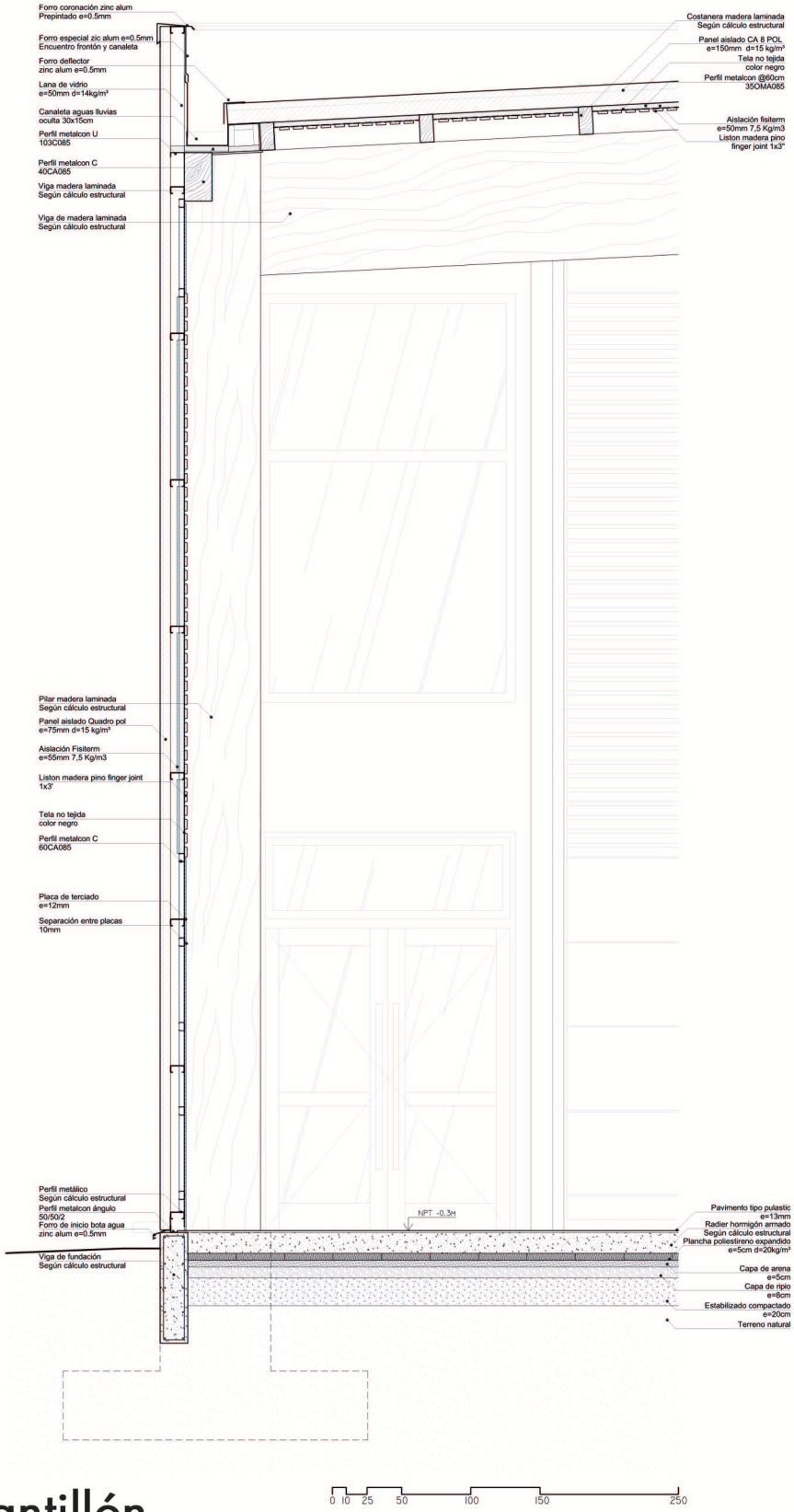
escantillón
