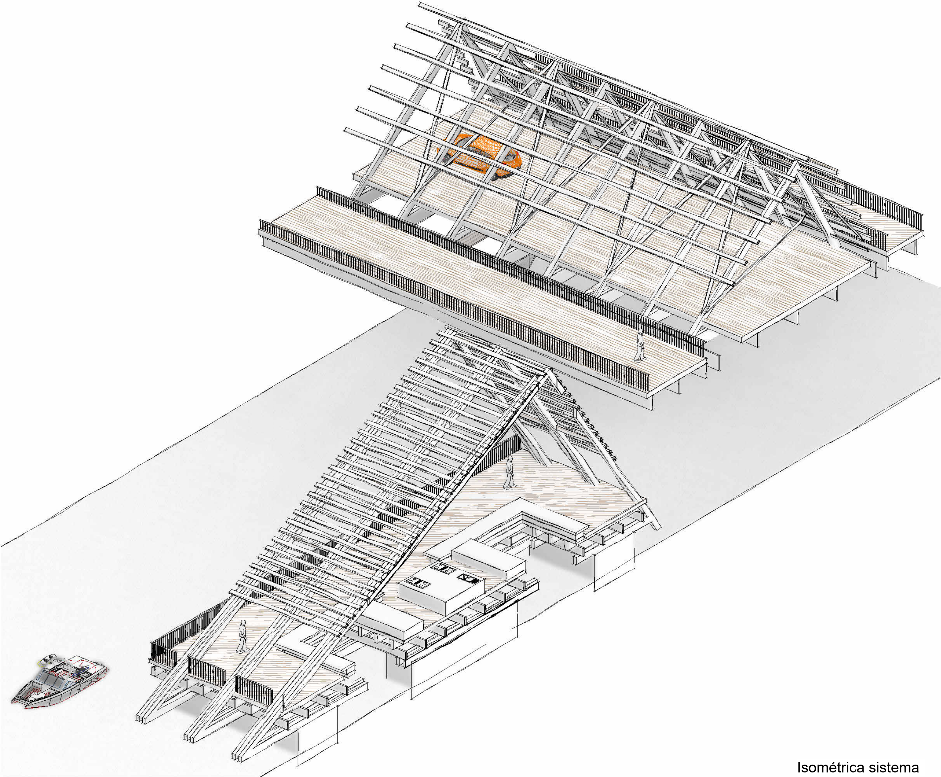
Isométrica sistema estructural 1:50
