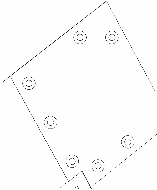
Pletina de acero inoxidable y pernos de acero para union con madera
