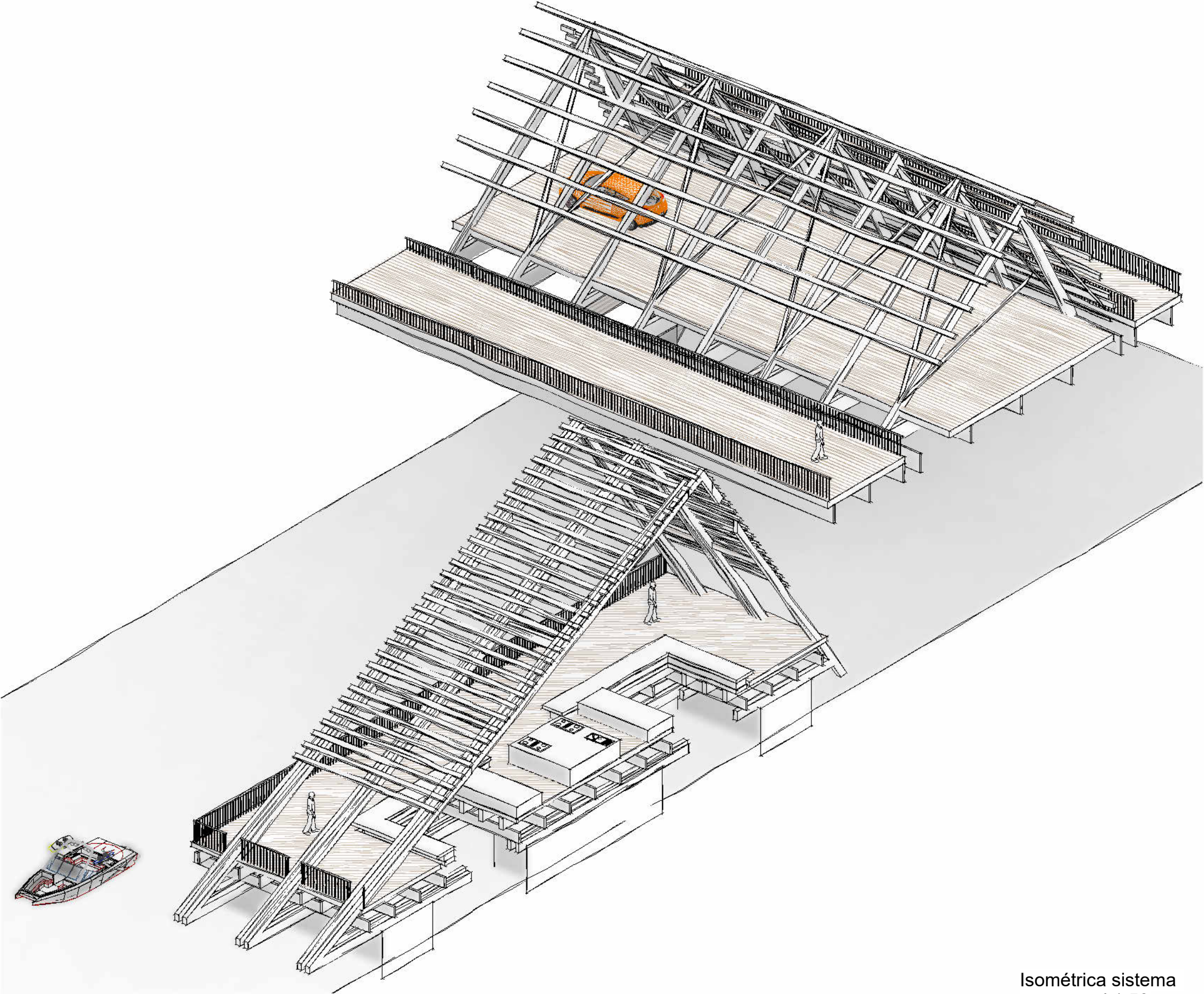
Isométrica sistema estructural 1:50
