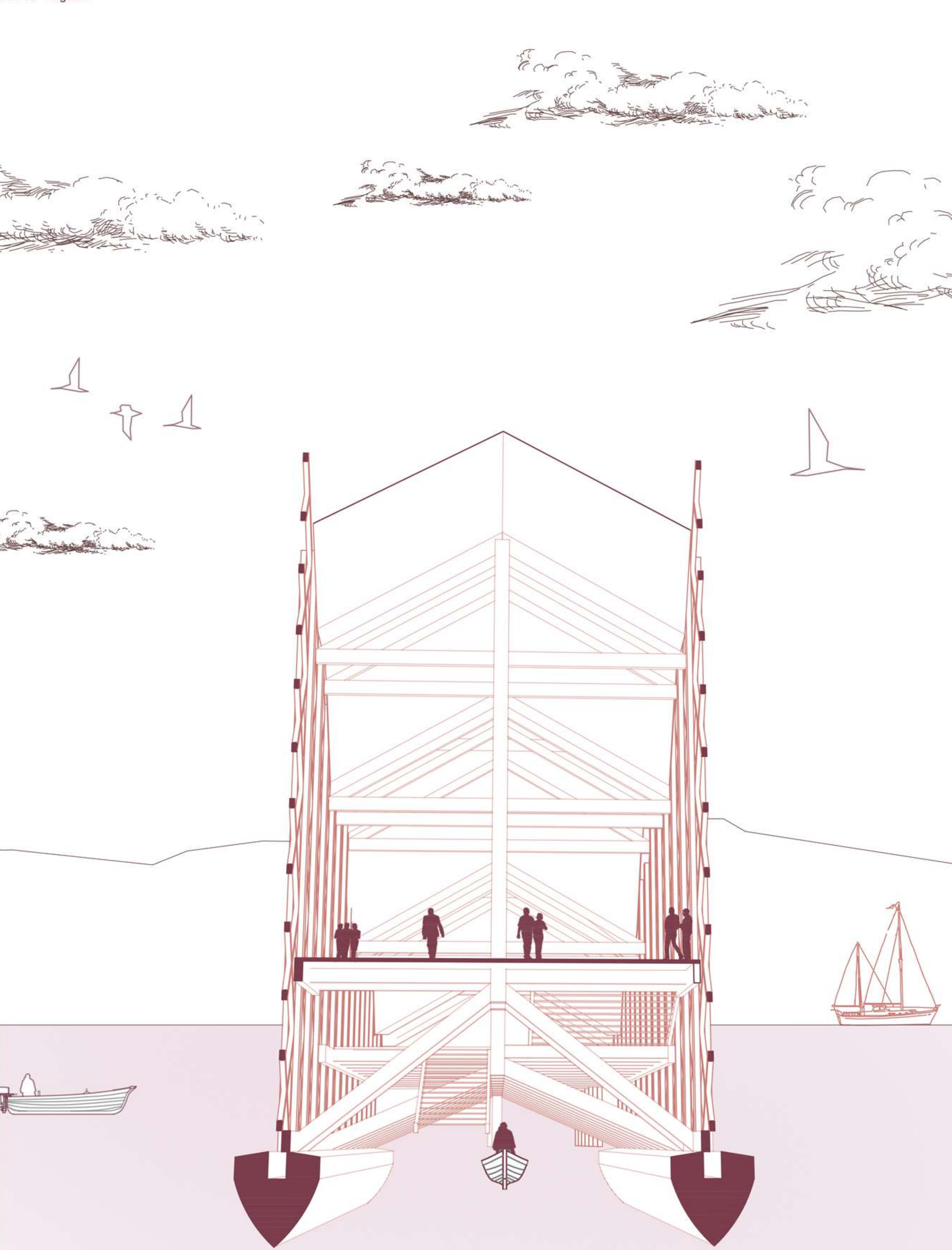
Corte fugado
