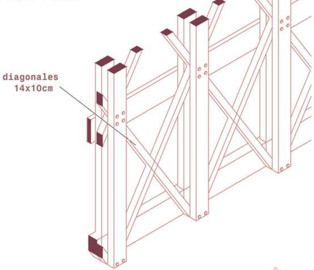
Corte detalle flotadores Flotadores de 150cm x 80cm
