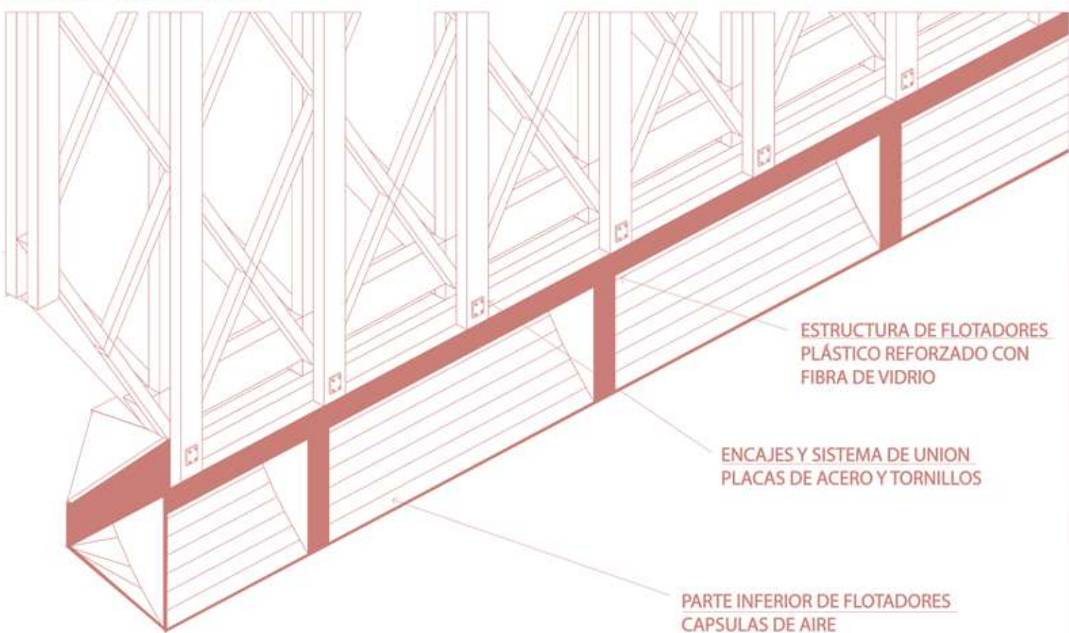
Detalle flotadores
