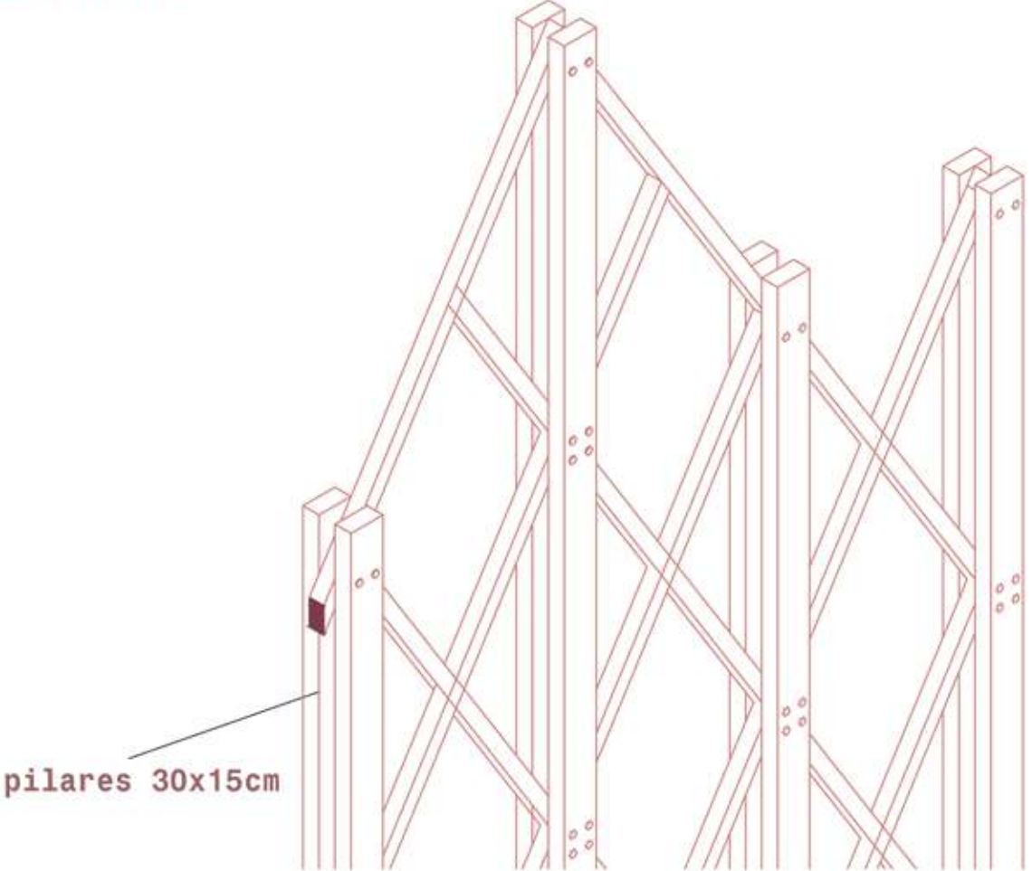
Detalle cercha
