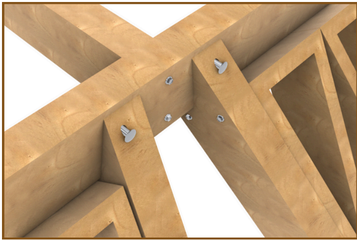
Unión de vigas con perno coche al techo
