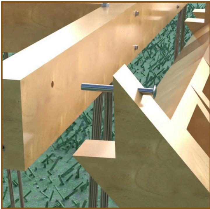
Boca de pescado con perno coche
