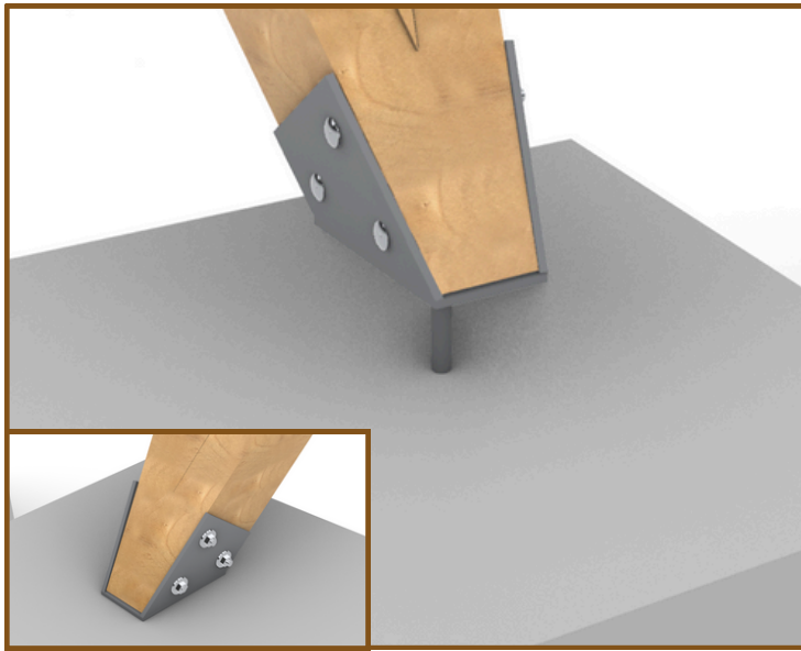
Pernos coche y fierro liso enterrado al hormigón
