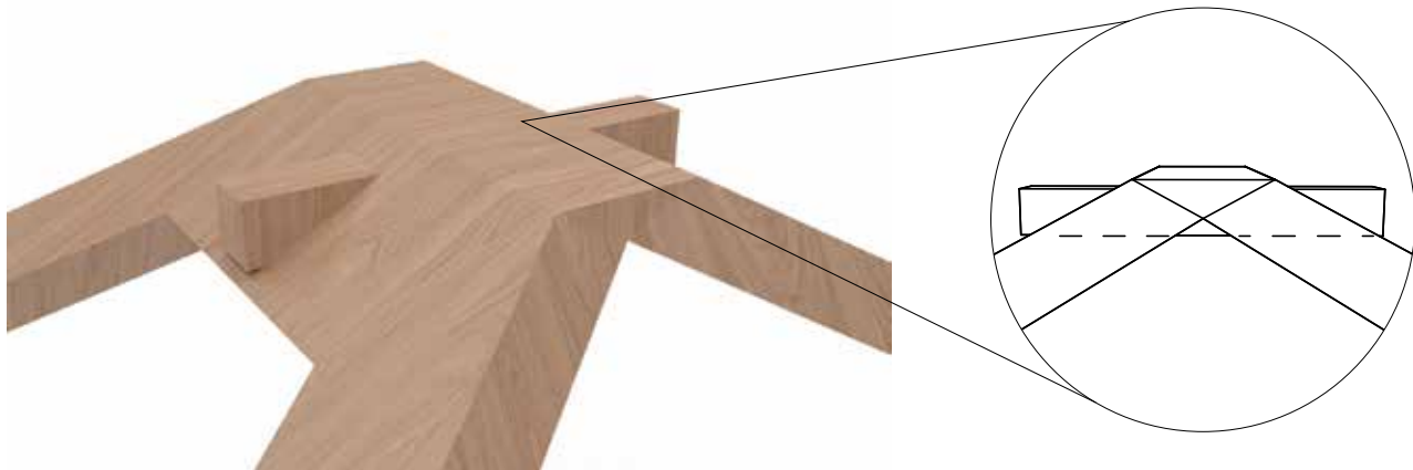
Las formas octogonales del techo se unen mediante el paso de un listón de madera mediante ensamble.
