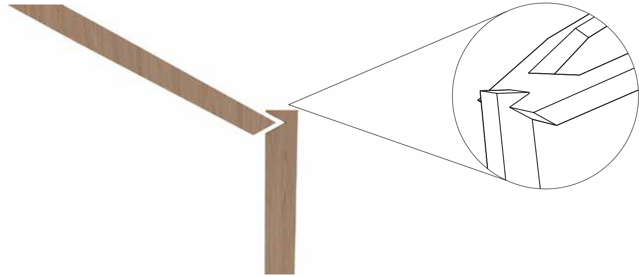
Unión de octágonos con listones mediante encaje.
