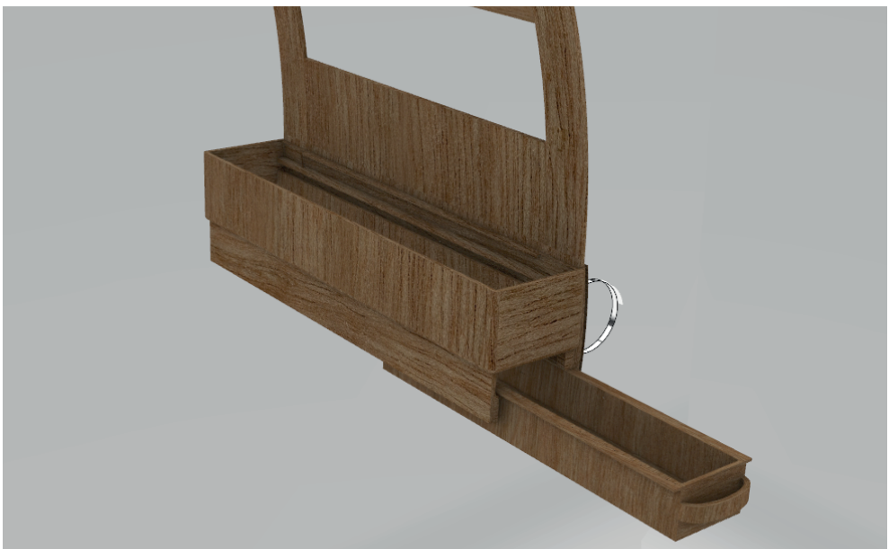
Sujeción a baranda de pasarela y orificios en el modulo mediante Zuncho metálico
